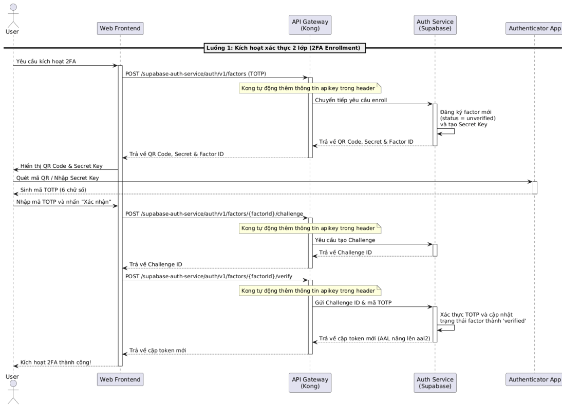
Hình 1.13: Sơ đồ tuần tự luồng Kích hoạt xác thực 2 lớp
