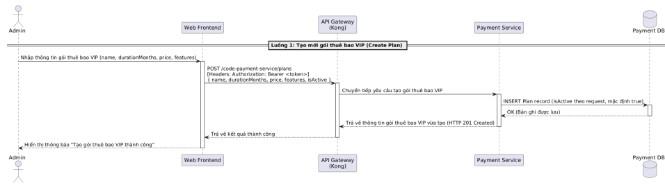
Hình 1.30: Sơ đồ tuần tự luồng Tạo mới gói thuê bao VIP
