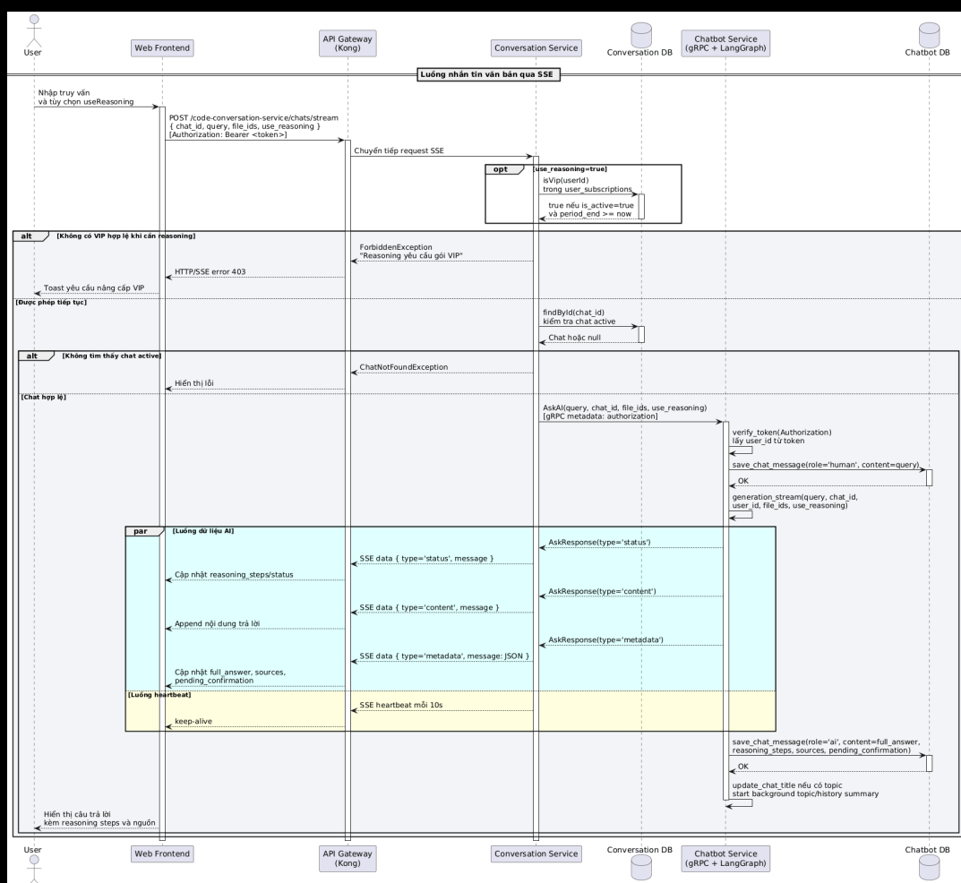
Hình 1.23: Sơ đồ tuần tự luồng nhấn tin văn bản qua SSE
