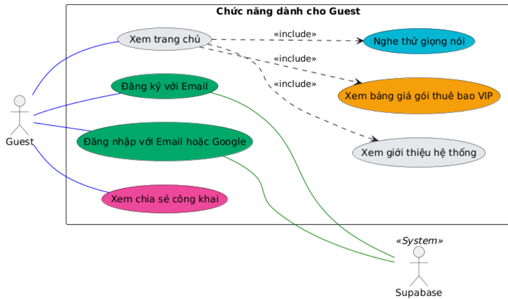
Hình 1.3: Sơ đồ Use Case - Guest
