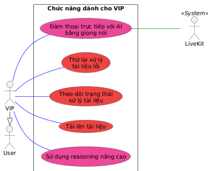
Hình 1.6: Sơ đồ Use Case - VIP
