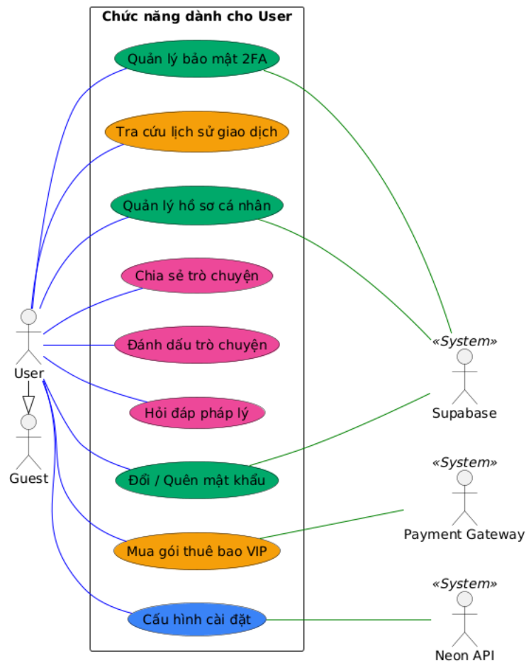
Hình 1.4: Sơ đồ Use Case - User
