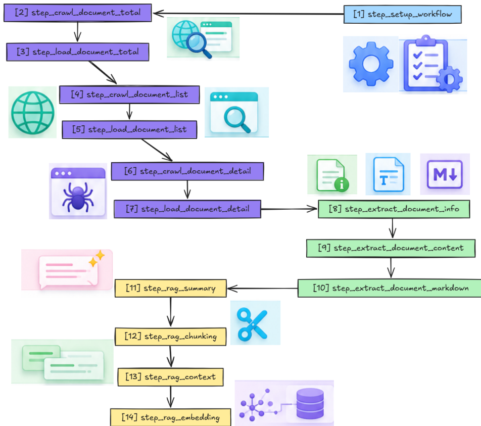
Hình 0.9: Sơ đồ các bước thực hiện của quy trình cũ
