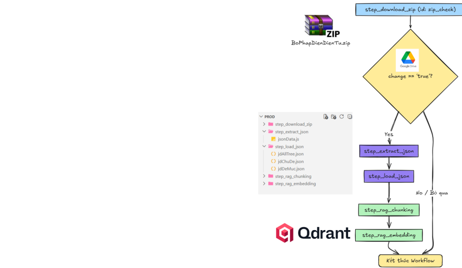
Hình 0.28: Sơ đồ thu thập dữ liệu chung
