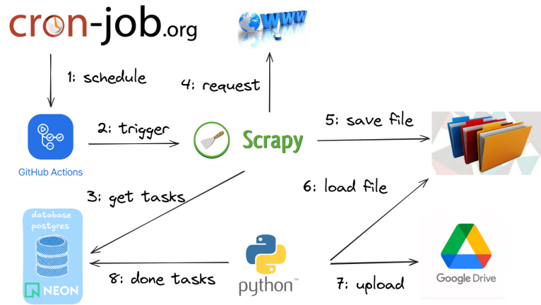
Hình 0.3: Sơ đồ thu thập dữ liệu chung
