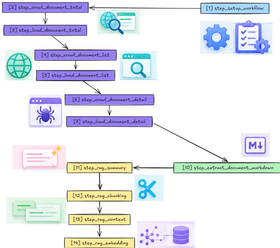
Hình 0.19: Sơ đồ các bước thực hiện của quy trình mới
