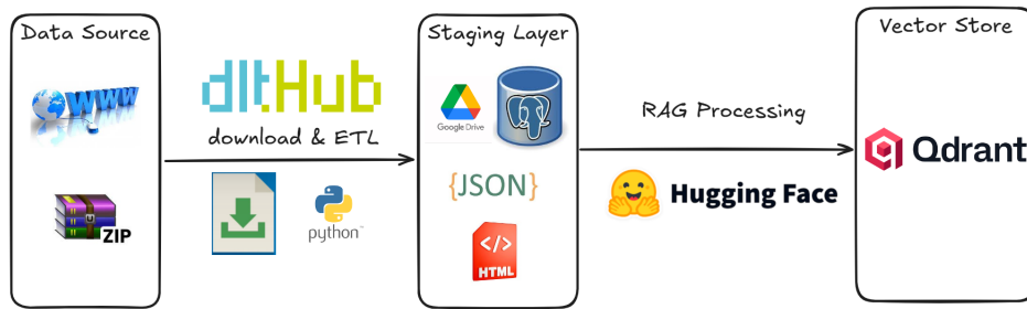
Hình 0.24: Sơ đồ thu thập dữ liệu chung
