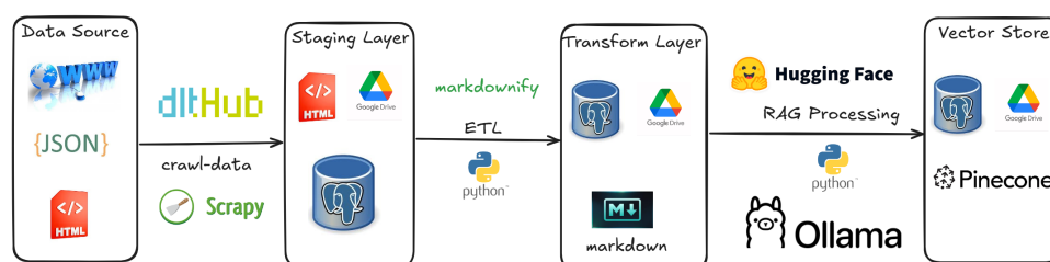
Hình 0.8: Sơ đồ tổng quan Data pipeline Văn bản pháp luật mới
