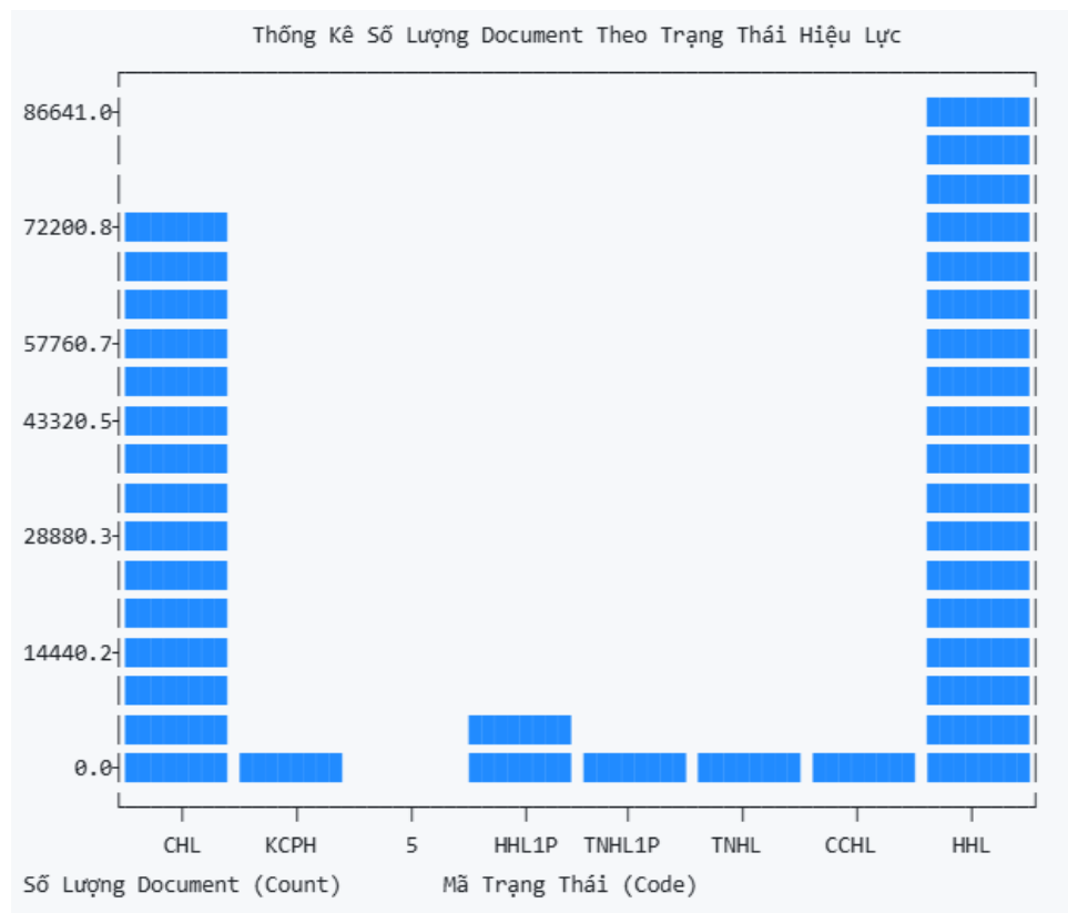
Hình 0.23: Kết quả chạy thành công các bước của Data Pipeline mới (Phần 3)
