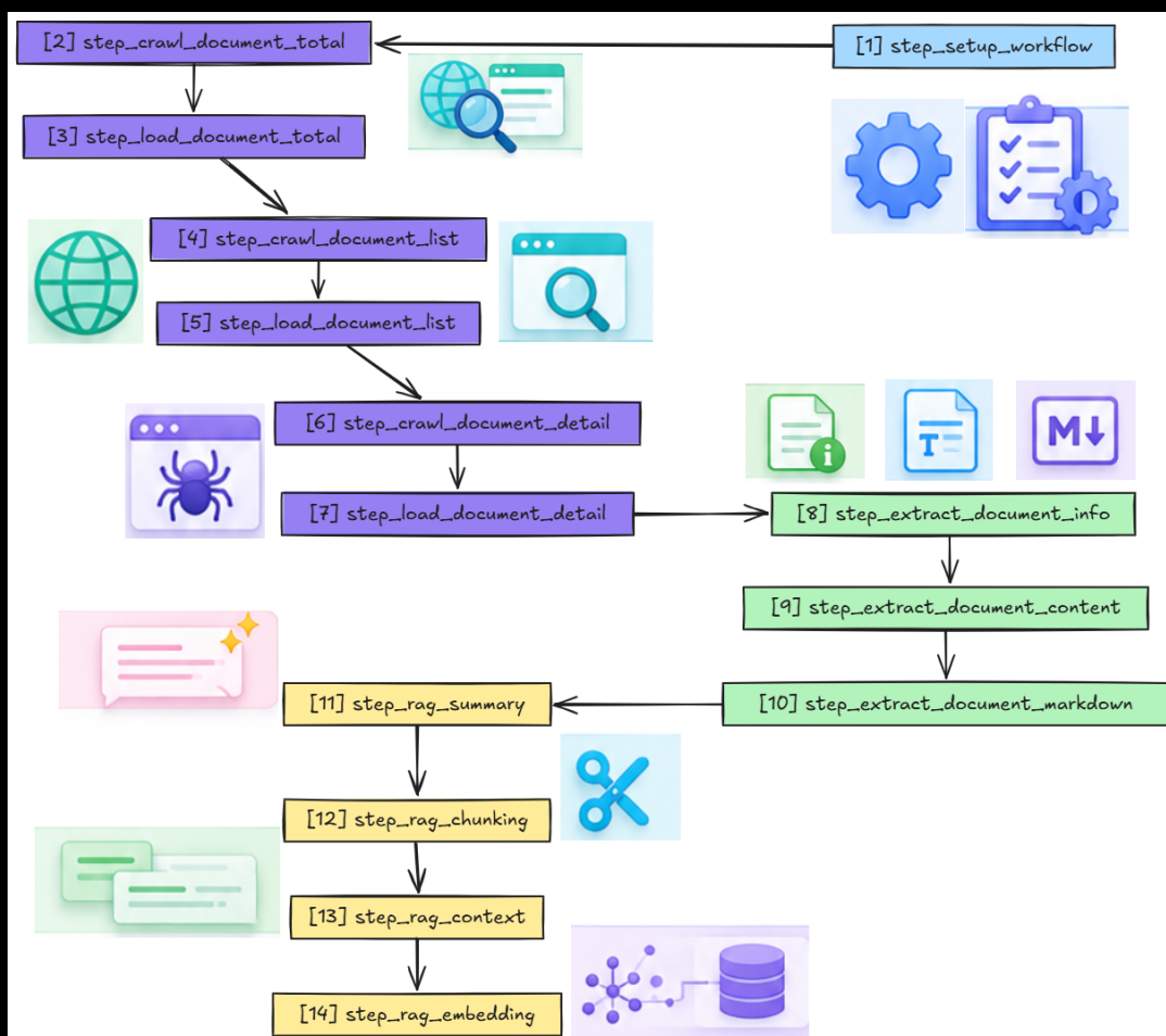
Hình 0.3: Sơ đồ các bước thực hiện của quy trình cũ
