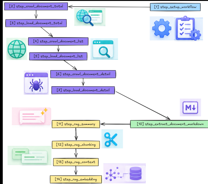
Hình 0.13: Sơ đồ các bước thực hiện của quy trình mới
