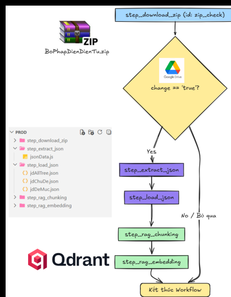
Hình 0.21: Sơ đồ thu thập dữ liệu chung
