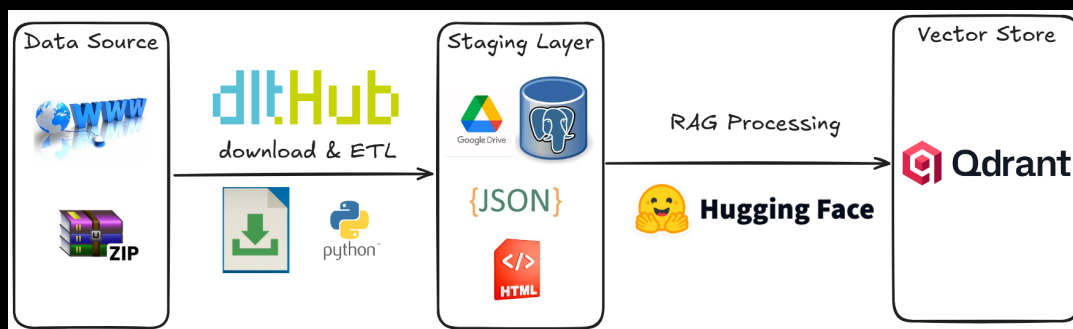
Hình 0.17: Sơ đồ thu thập dữ liệu chung
