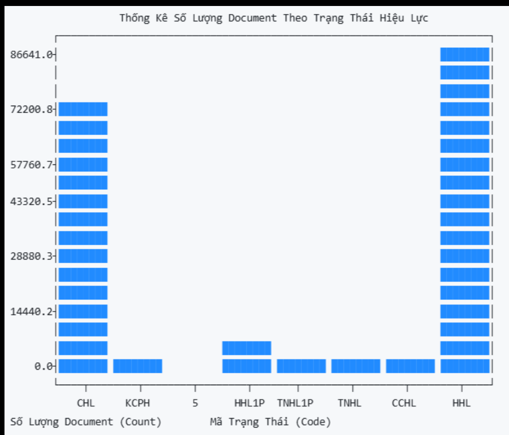
Hình 0.16: Kết quả chạy các bước luồng dữ liệu VBPL mới (Phần 3)
