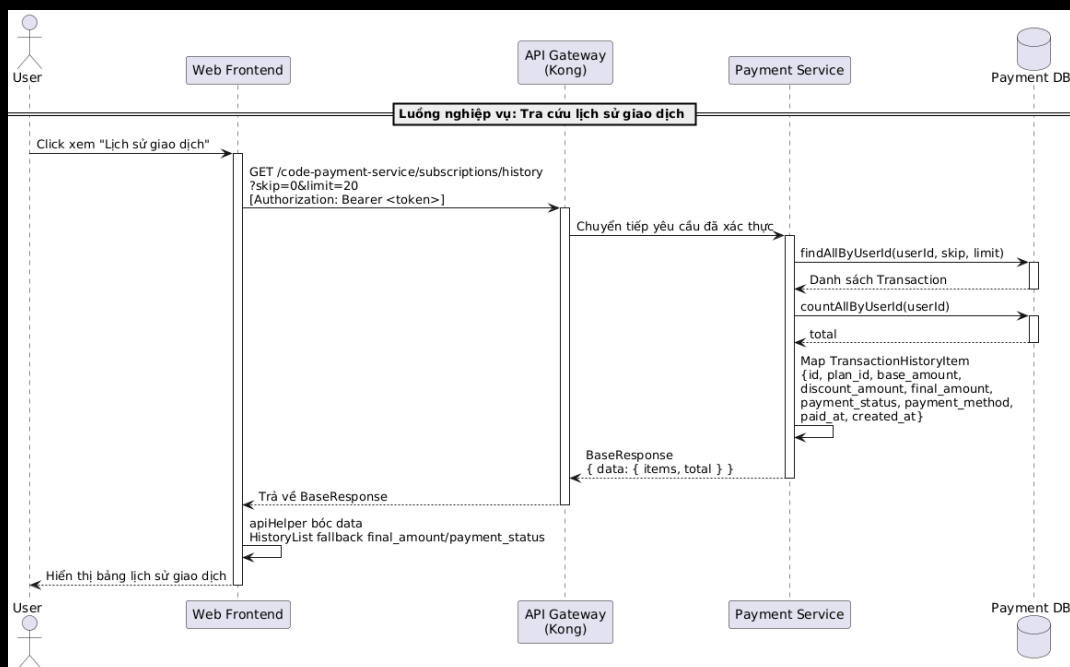
Hình 1.40: Sơ đồ tuần tự luồng tra cứu lịch sử giao dịch
