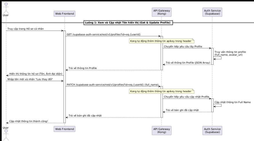
Hình 1.16: Sơ đồ tuần tự luồng Xem và Cập nhật Tên hiển thị
