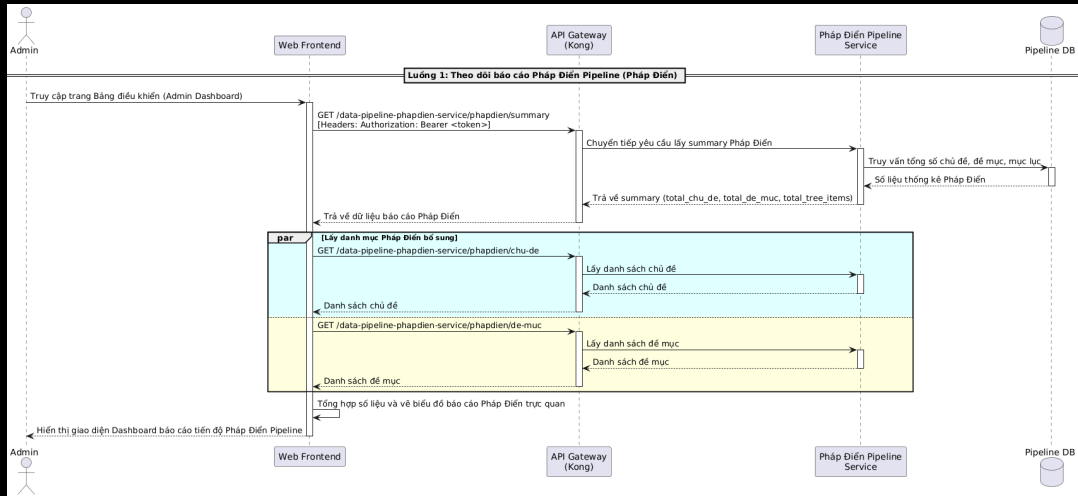
Hình 1.32: Sơ đồ tuần tự luồng Theo dõi báo cáo Pháp Diễn Pipeline
