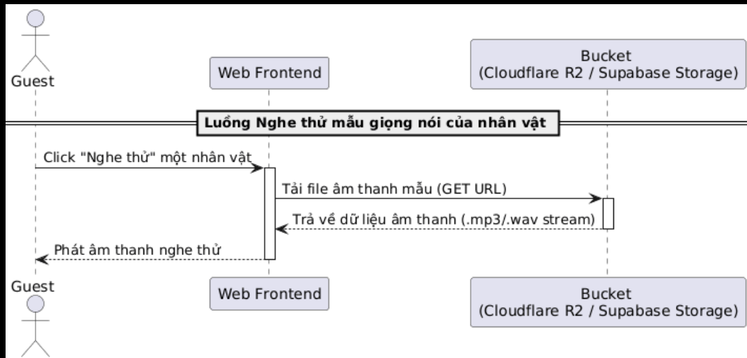
Hình 1.8: Sơ đồ tuần tự luồng nghe thử mẫu giọng nói
