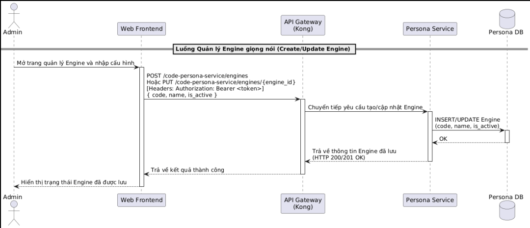
Hình 1.34: Sơ đồ tuần tự luồng Quản lý Engine giọng nói
