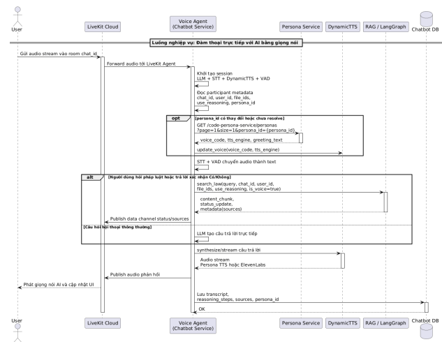
Hình 0.2: Sơ đồ tuần tự luồng Đàm thoại trực tiếp với AI bằng giọng nói
