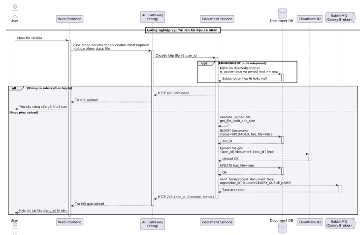
Hình 0.3: Sơ đồ tuần tự luồng Tải lên tài liệu cá nhân
