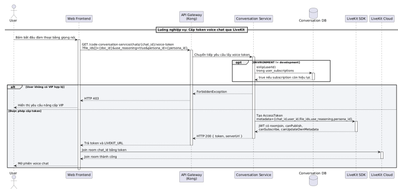
Hình 0.1: Sơ đồ tuần tự luồng Cấp token voice chat qua LiveKit
