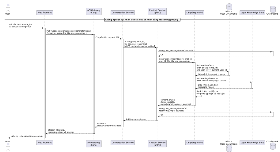
Hình 0.5: Sơ đồ tuần tự luồng Phân tích tài liệu cá nhân bằng reasoning pháp lý
