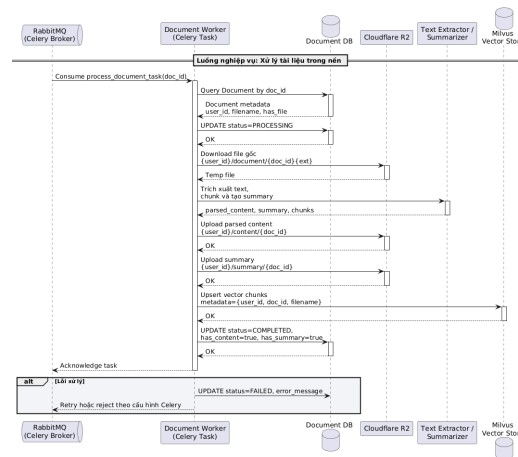
Hình 0.4: Sơ đồ tuần tự luồng Xử lý tài liệu trong nền
