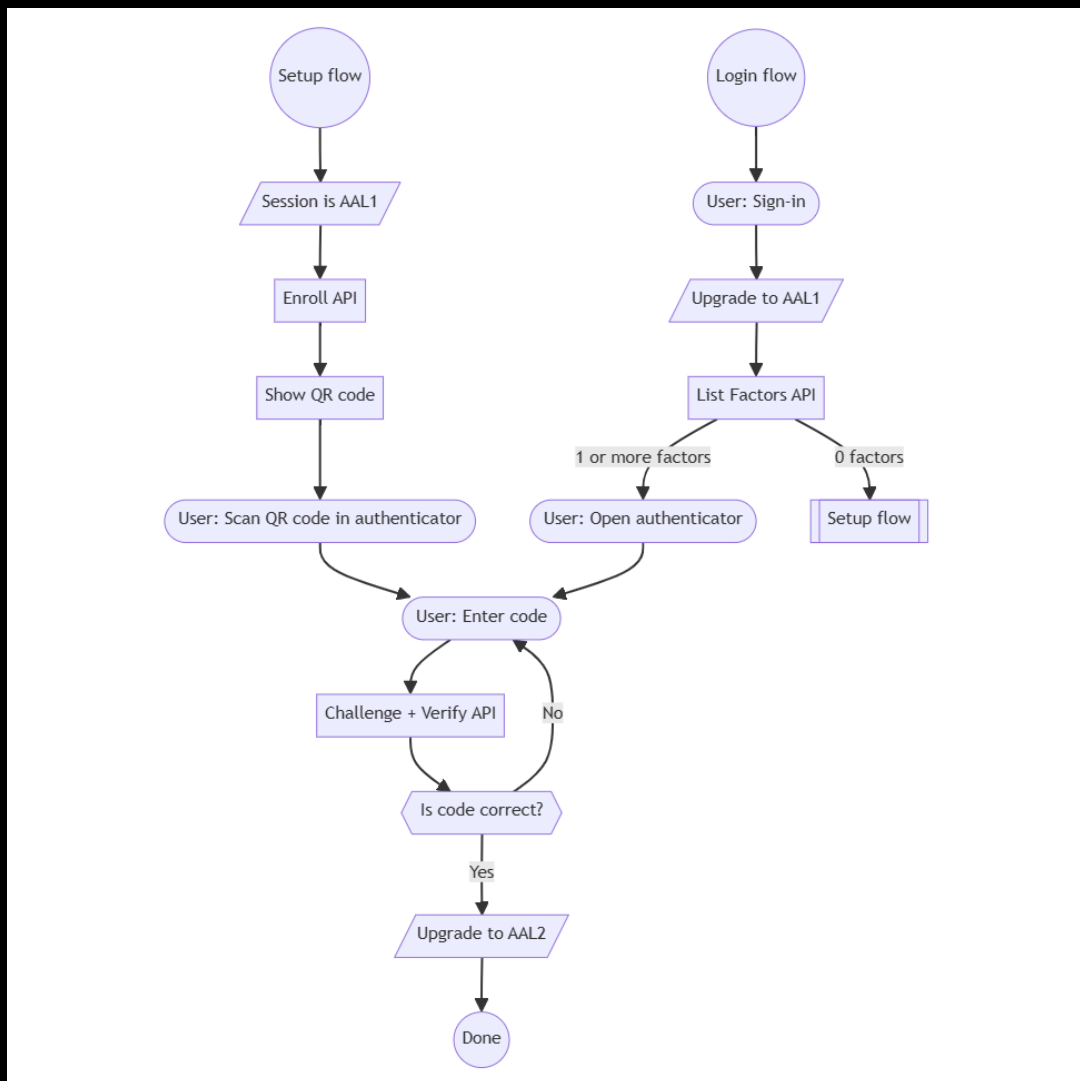
Hình 1.5: Sơ đồ luồng xử lý xác thực MFA
