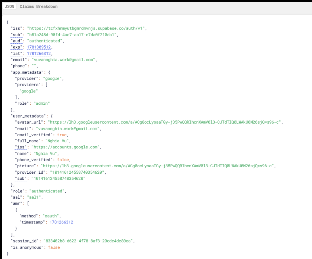
Hình 1.2: Thông tin JWT Payload từ Supabase
