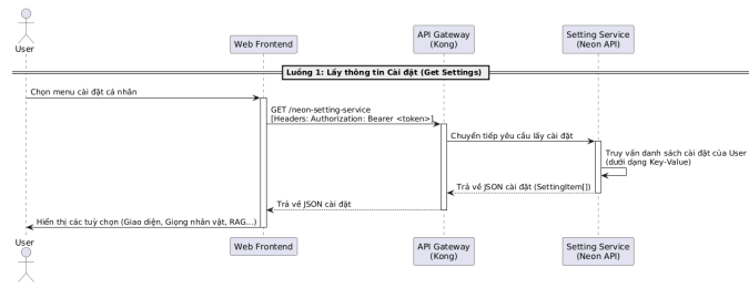
Hình 0.15: Sơ đồ tuần tự luồng Lấy thông tin Cài đặt
