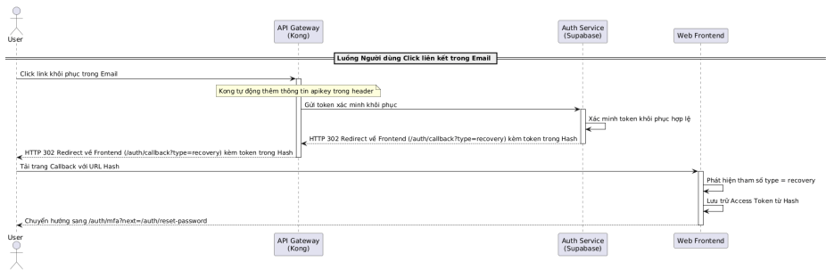
Hình 0.13: Sơ đồ tuần tự luồng Xác nhận liên kết từ Email
