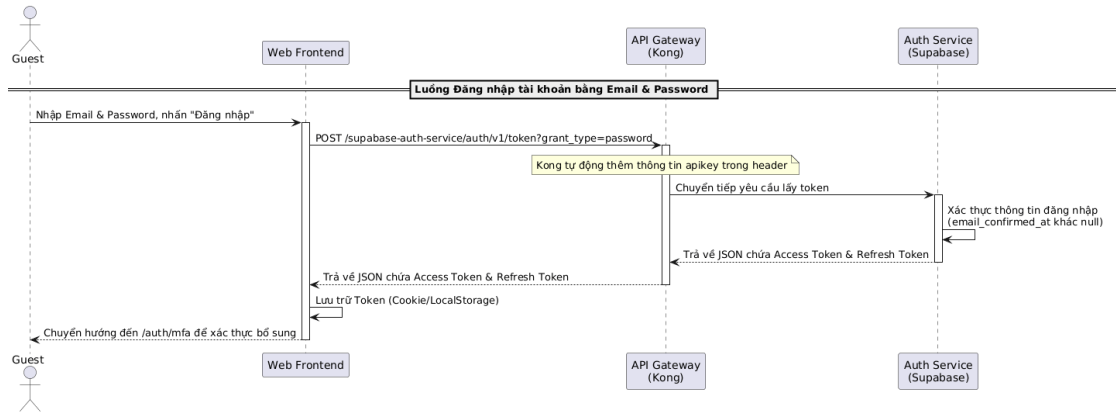
Hình 0.6: Sơ đồ tuần tự luồng đăng nhập bằng email & password
