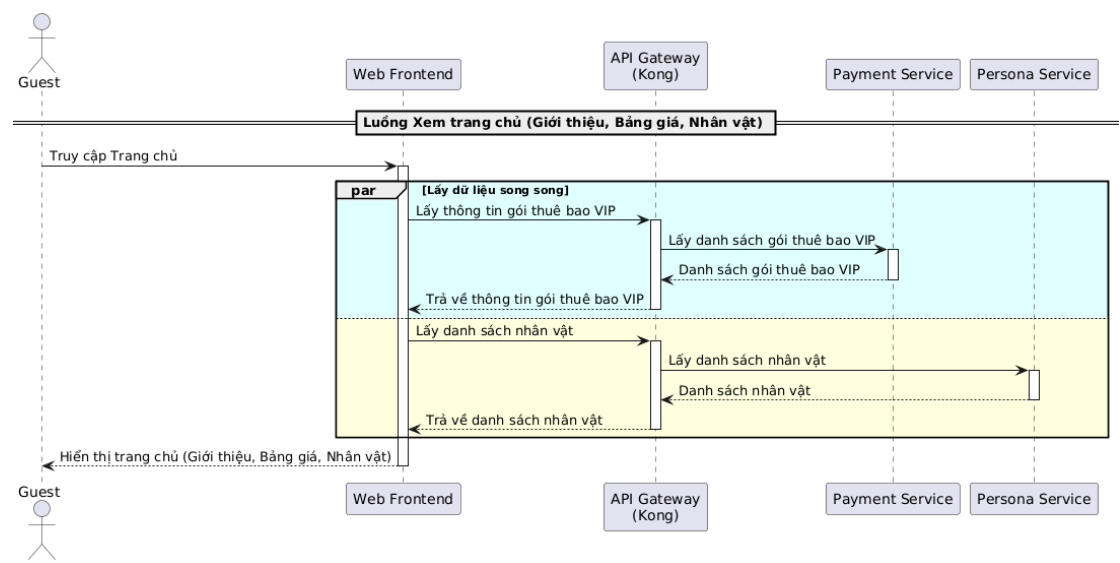
Hình 0.1: Sơ đồ tuần tự luồng xem trang chủ
