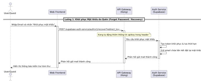
Hình 0.12: Sơ đồ tuần tự luồng Yêu cầu Khôi phục Mật khẩu
