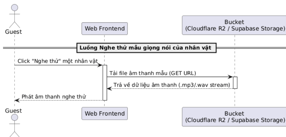
Hình 0.2: Sơ đồ tuần tự luồng nghe thử mẫu giọng nói
