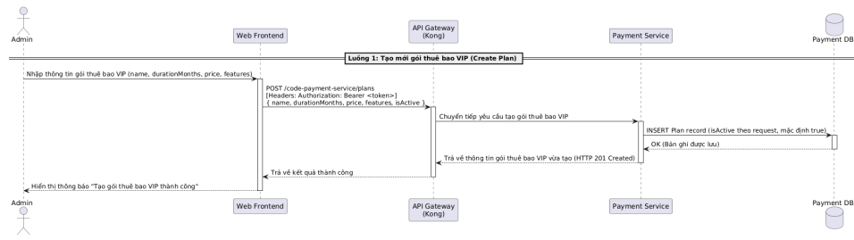
Hình 0.24: Sơ đồ tuần tự luồng Tạo mới gói thuê bao VIP
