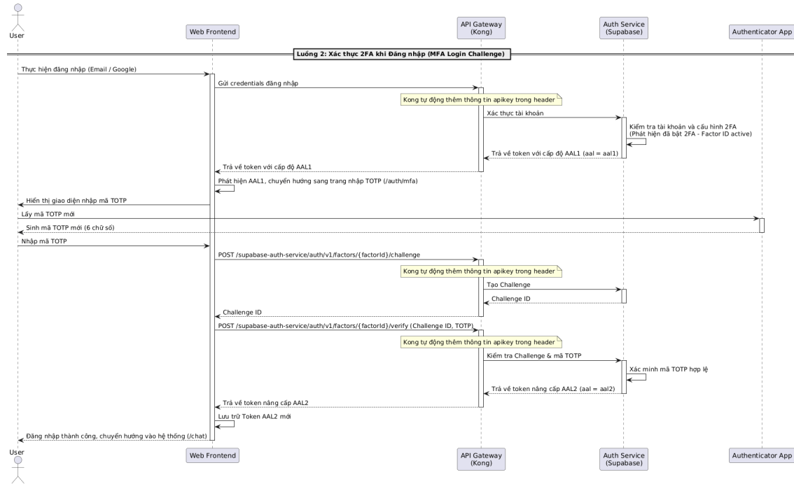
Hình 0.8: Sơ đồ tuần tự luồng Bắt buộc xác thực 2FA khi Đăng nhập
