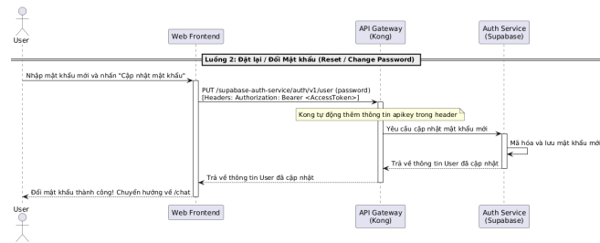
Hình 0.14: Sơ đồ tuần tự luồng Đặt lại / Đổi Mật khẩu
