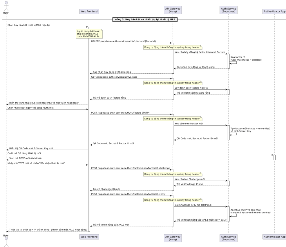
Hình 0.9: Sơ đồ tuần tự luồng Hủy liên kết và thiết lập lại thiết bị MFA
