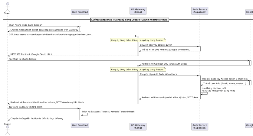
Hình 0.3: Sơ đồ tuần tự luồng Đăng nhập / Đăng ký bằng Google
