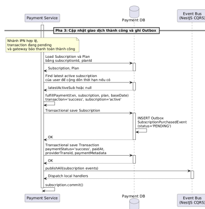
Hình 0.31: Sơ đồ tuần tự luồng cập nhật giao dịch thành công và ghi Outbox
