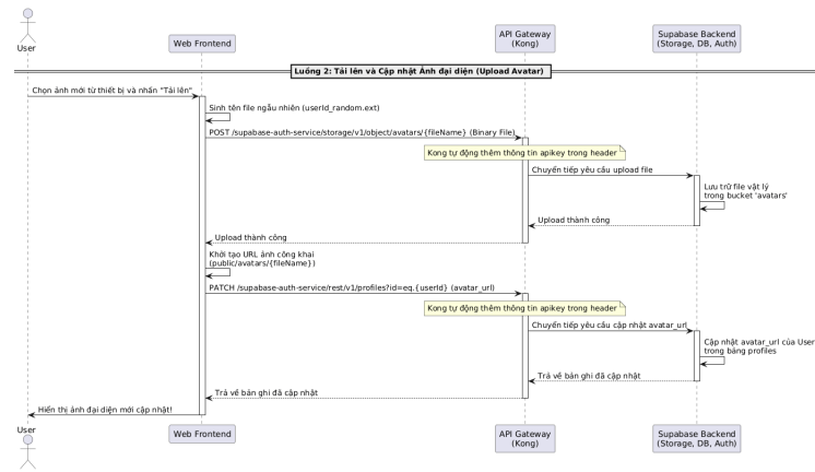
Hình 0.11: Sơ đồ tuần tự luồng Tải lên và Cập nhật Ảnh đại diện
