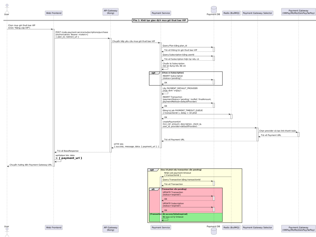
Hình 0.29: Sơ đồ tuần tự luồng khởi tạo giao dịch mua gói thuê bao VIP
