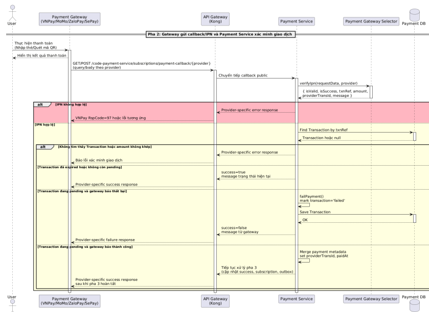
Hình 0.30: Sơ đồ tuần tự luồng cổng thanh toán gửi IPN và dịch vụ thanh toán xác minh giao dịch
