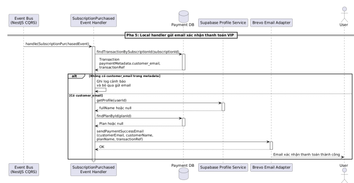
Hình 0.33: Sơ đồ tuần tự luồng gửi email xác nhận thanh toán VIP
