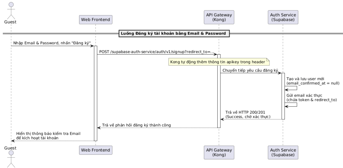
Hình 0.4: Sơ đồ tuần tự luồng đăng ký tài khoản bằng email
