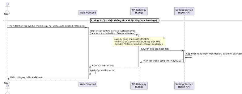
Hình 0.16: Sơ đồ tuần tự luồng Cập nhật thông tin Cài đặt
