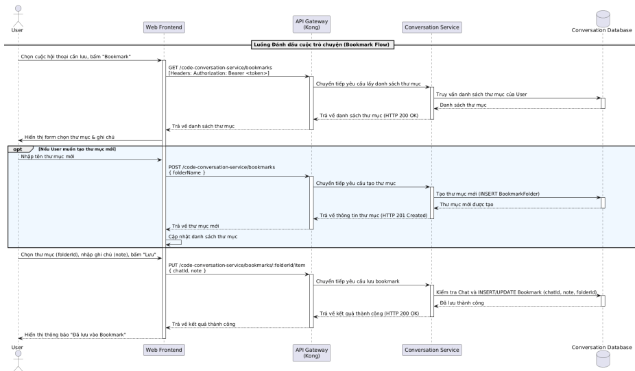
Hình 0.21: Sơ đồ tuần tự luồng Đánh dấu cuộc trò chuyện
