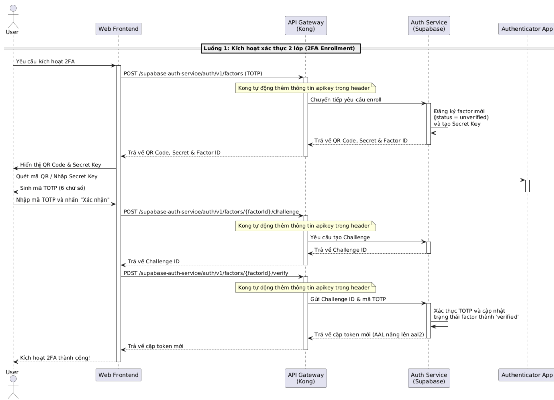
Hình 0.7: Sơ đồ tuần tự luồng Kích hoạt xác thực 2 lớp
