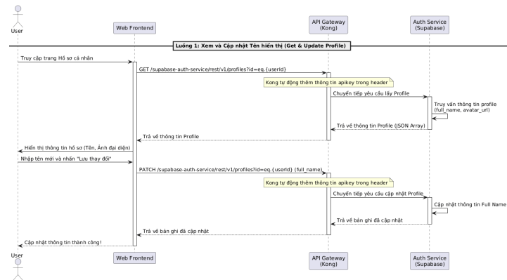
Hình 0.10: Sơ đồ tuần tự luồng Xem và Cập nhật Tên hiển thị
