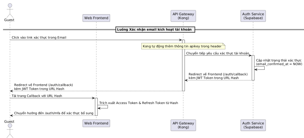
Hình 0.5: Sơ đồ tuần tự luồng Xác nhận Email kích hoạt tài khoản
