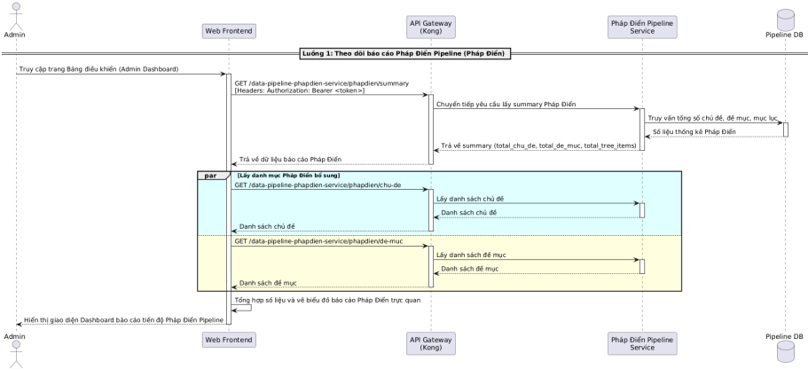
Hình 0.26: Sơ đồ tuần tự luồng Theo dõi báo cáo Pháp Diễn Pipeline
