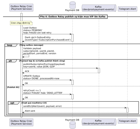
Hình 0.32: Sơ đồ tuần tự luồng Outbox Relay xuất bản sự kiện mua VIP lên Kafka
