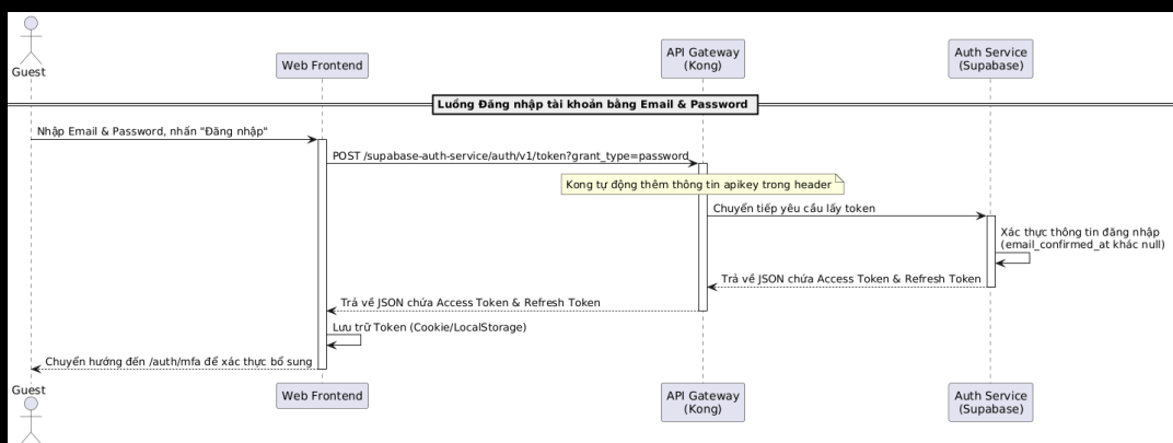
Hình 0.6: Sơ đồ tuần tự luồng đăng nhập bằng email & password
