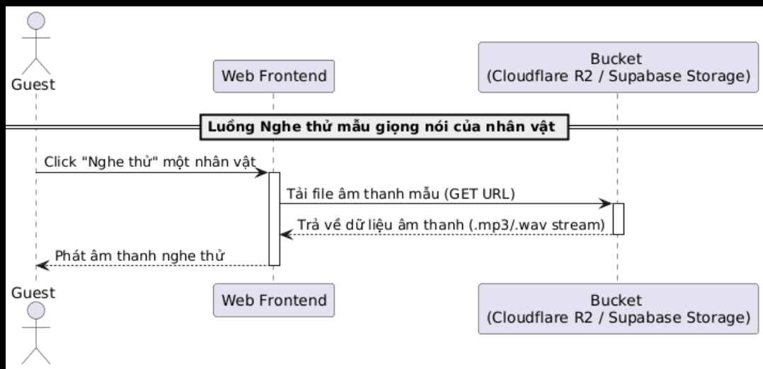
Hình 0.2: Sơ đồ tuần tự luồng nghe thử mẫu giọng nói của nhân vật
