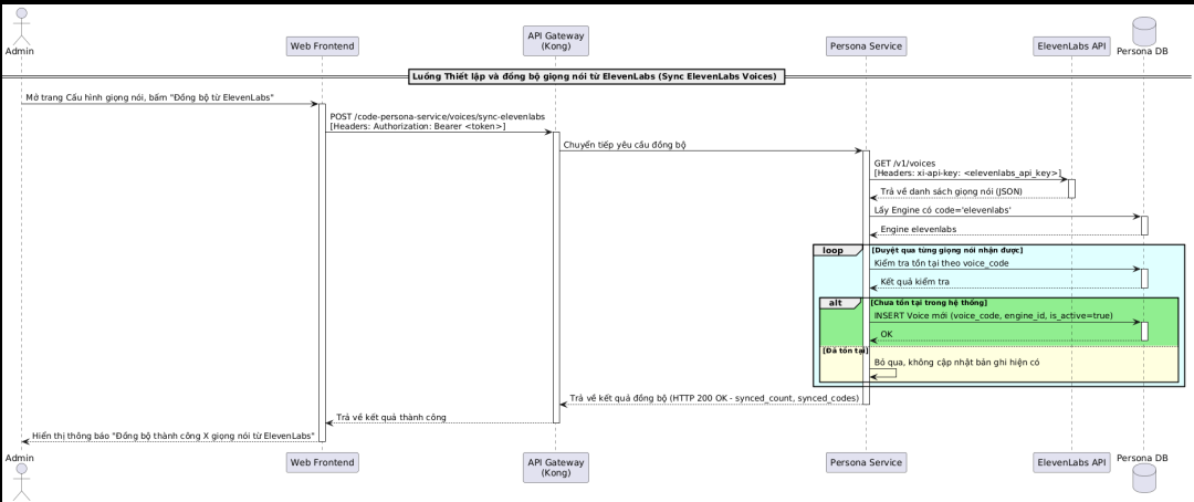
Hình 0.23: Sơ đồ tuần tự luồng thiết lập và đồng bộ giọng nói từ ElevenLabs
