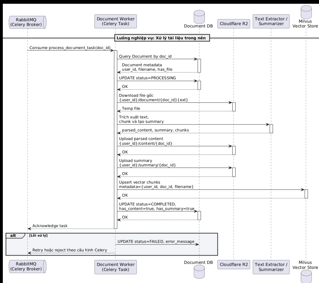
Hình 0.38: Sơ đồ tuần tự luồng xử lý tài liệu trong nền
