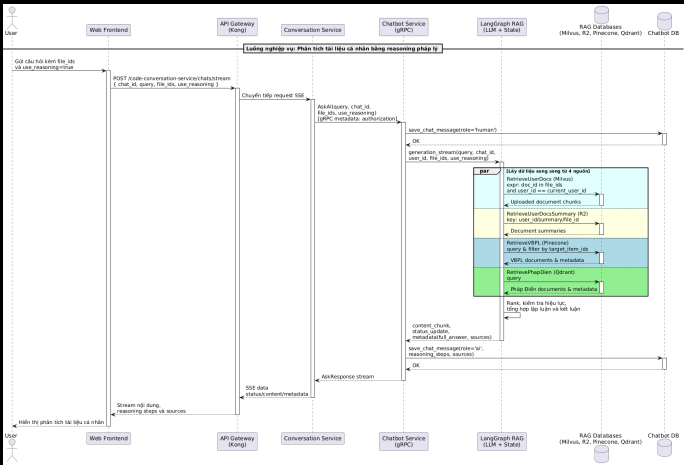
Hình 0.39: Sơ đồ tuần tự luồng phân tích tài liệu cá nhân bằng reasoning pháp lý
