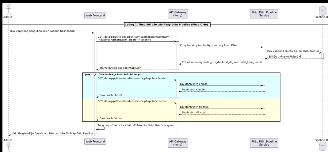
Hình 0.26: Sơ đồ tuần tự luồng theo dõi báo cáo pháp điển pipeline
