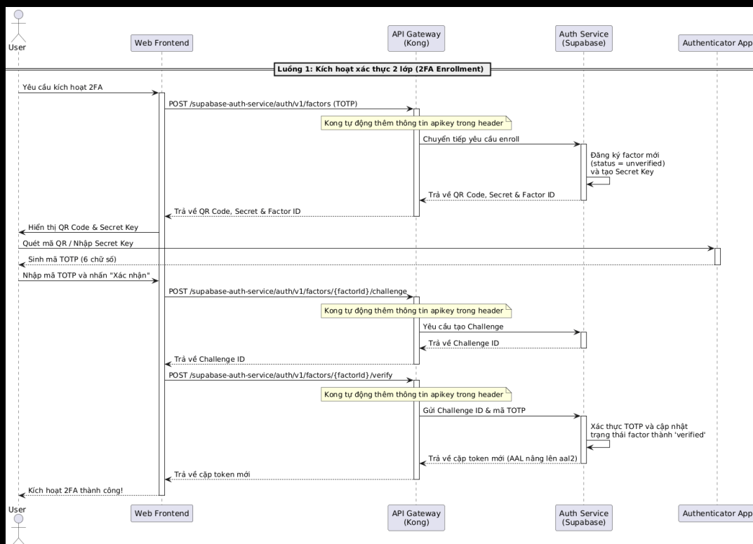
Hình 0.7: Sơ đồ tuần tự luồng kích hoạt xác thực 2 lớp
