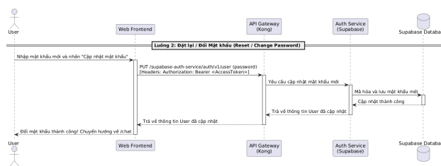
Hình 0.14: Sơ đồ tuần tự Đặt lại / Đổi Mật khẩu
