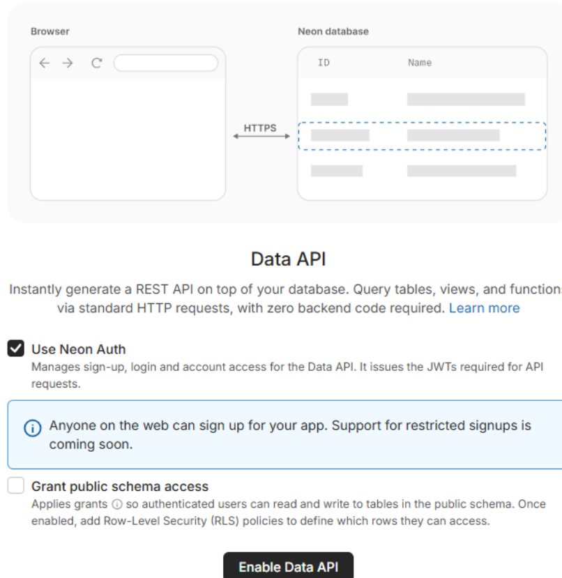
Hình 1.7: Kích hoạt Data API trên Neon
