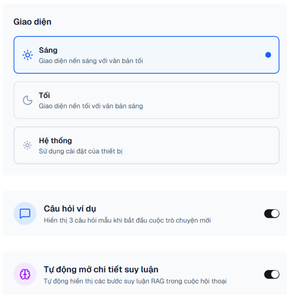
Hình 1.20: Cài đặt người dùng
