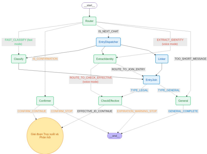
Hình 0.1: Sơ đồ LangGraph (Giai đoạn Tiếp nhận và Điều hướng)
