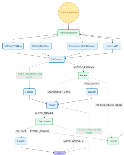
Hình 0.2: Sơ đồ LangGraph (Giai đoạn Truy xuất và Phản hồi)
