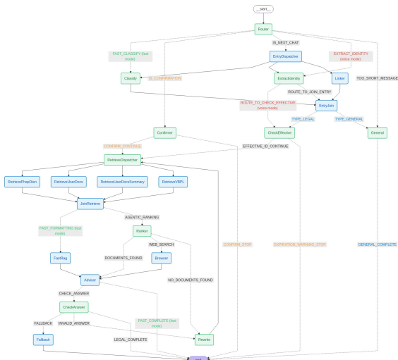
Hình 0.3: Sơ đồ LangGraph của dự án
