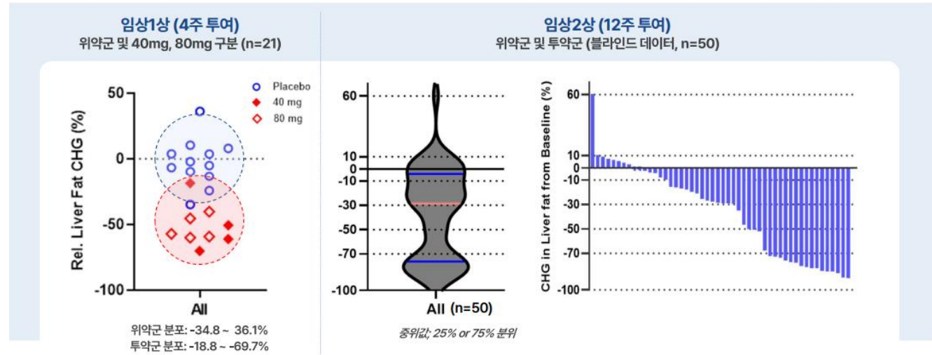
그림 2. DD01 임상 1상 및 임상 2상 지방간 감소 분포도
