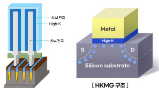
그림 10. High-K 기반 트랜지스터 구조 및 HKMG 개념도
