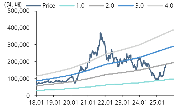
그림 2. P/B Band
