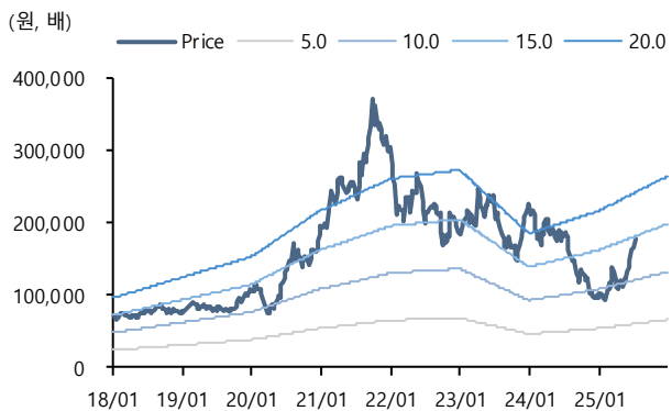
그림 1. P/E Band
