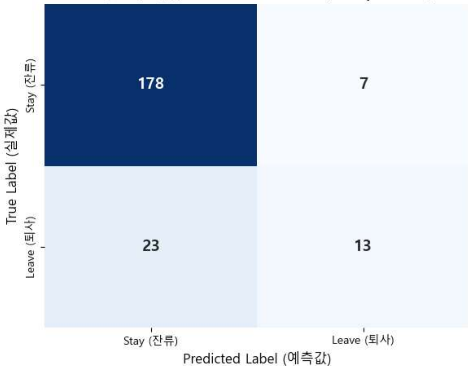
로지스틱 회귀 Confusion Matrix (Test | Th: 0.5)
