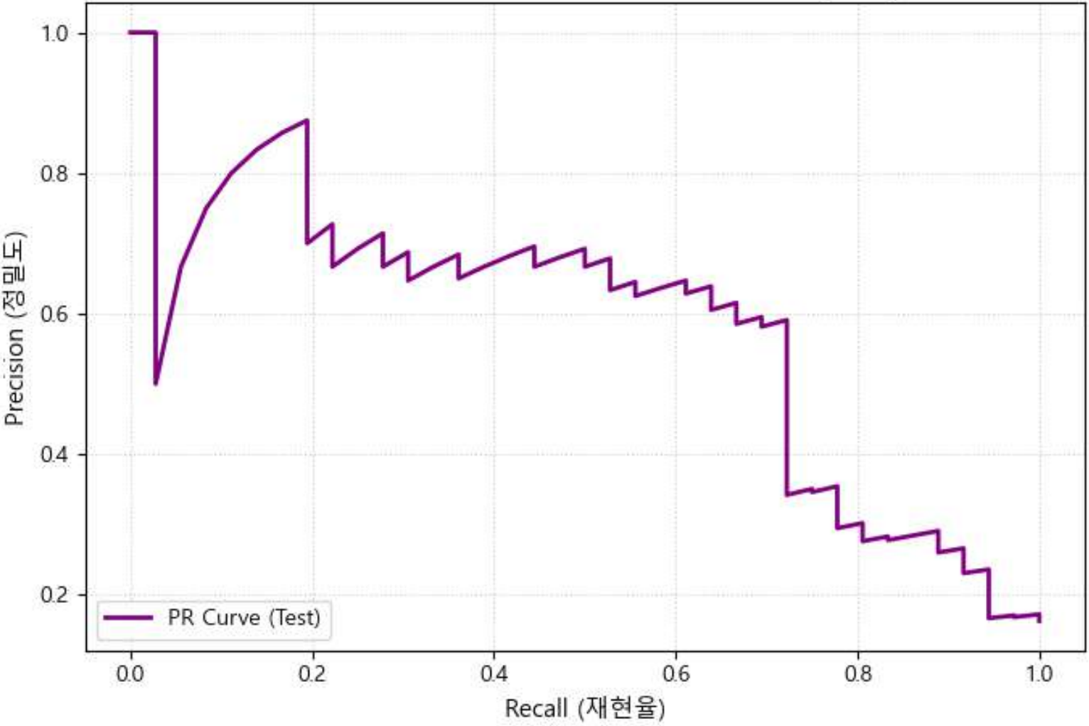
로지스틱 회귀 Precision-Recall Curve (Test)
