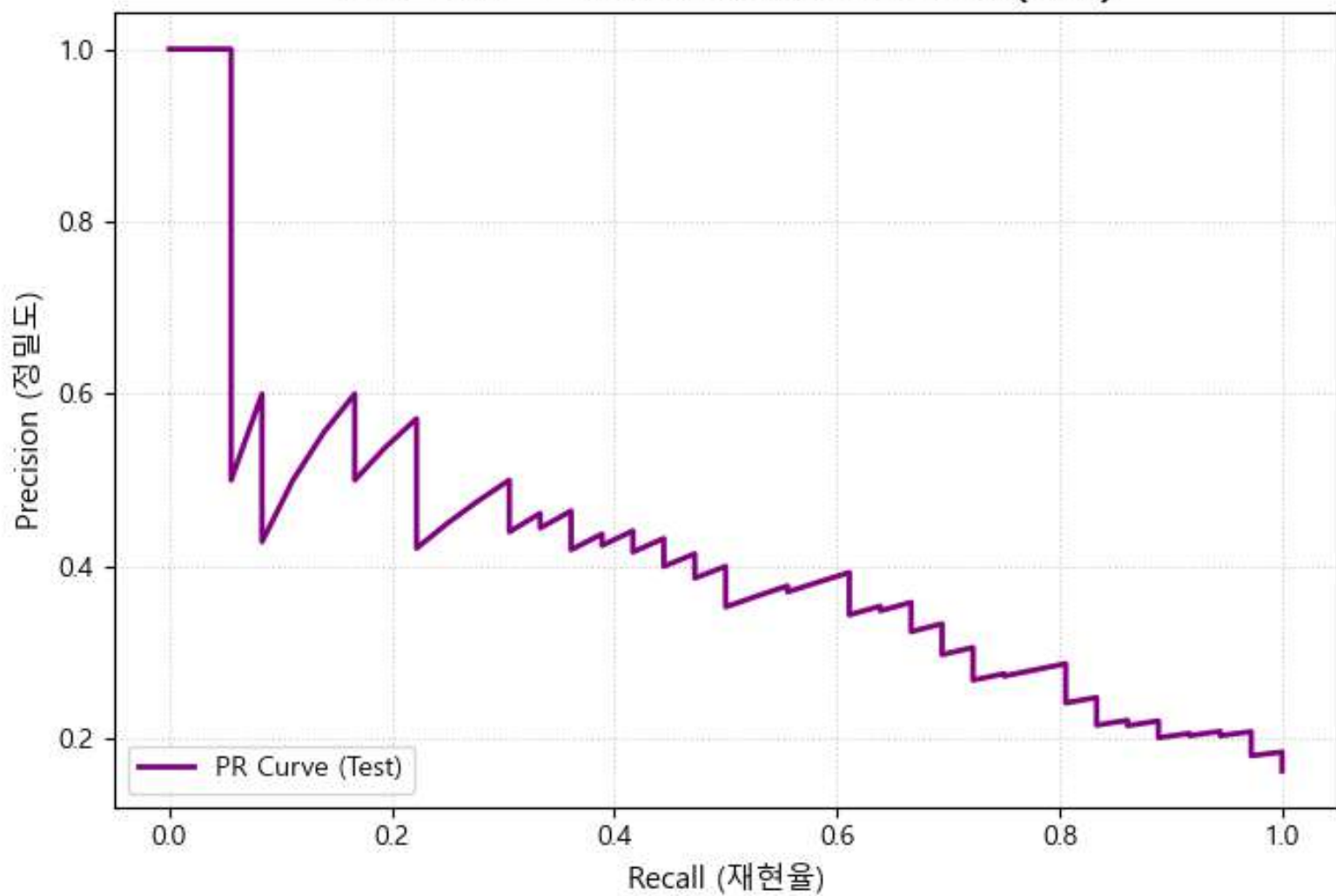
랜덤 포레스트 Precision-Recall Curve (Test)
