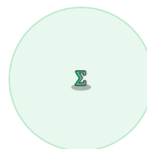
Helper
