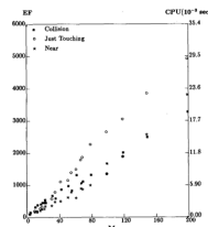
F13 计算复杂度和加速比图
