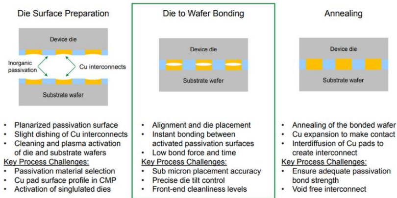
그림 4. Hybrid Bonding 공정의 전개
