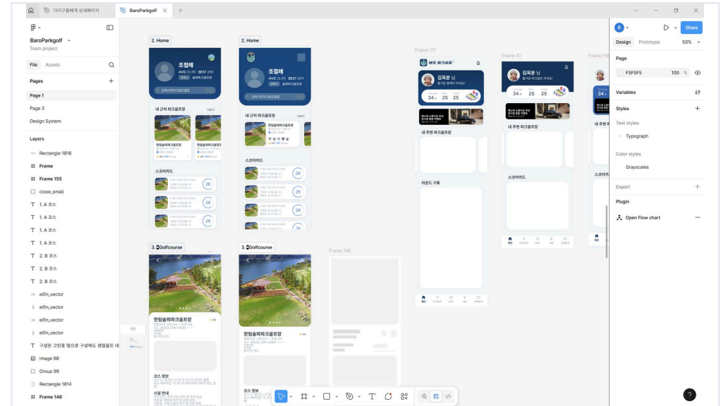
Figma 프로토타입
