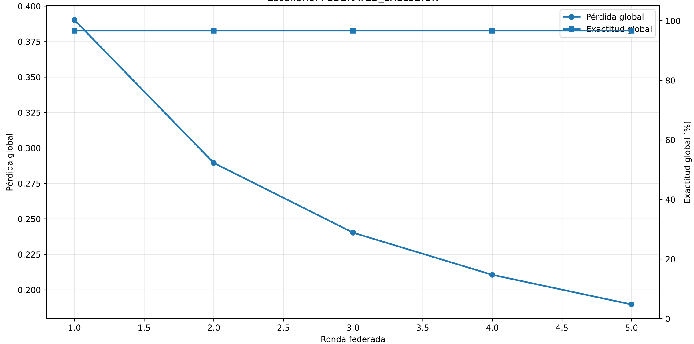
Aprendizaje federado FedAvg Escenario: FEDERATED_EXCLUSION
