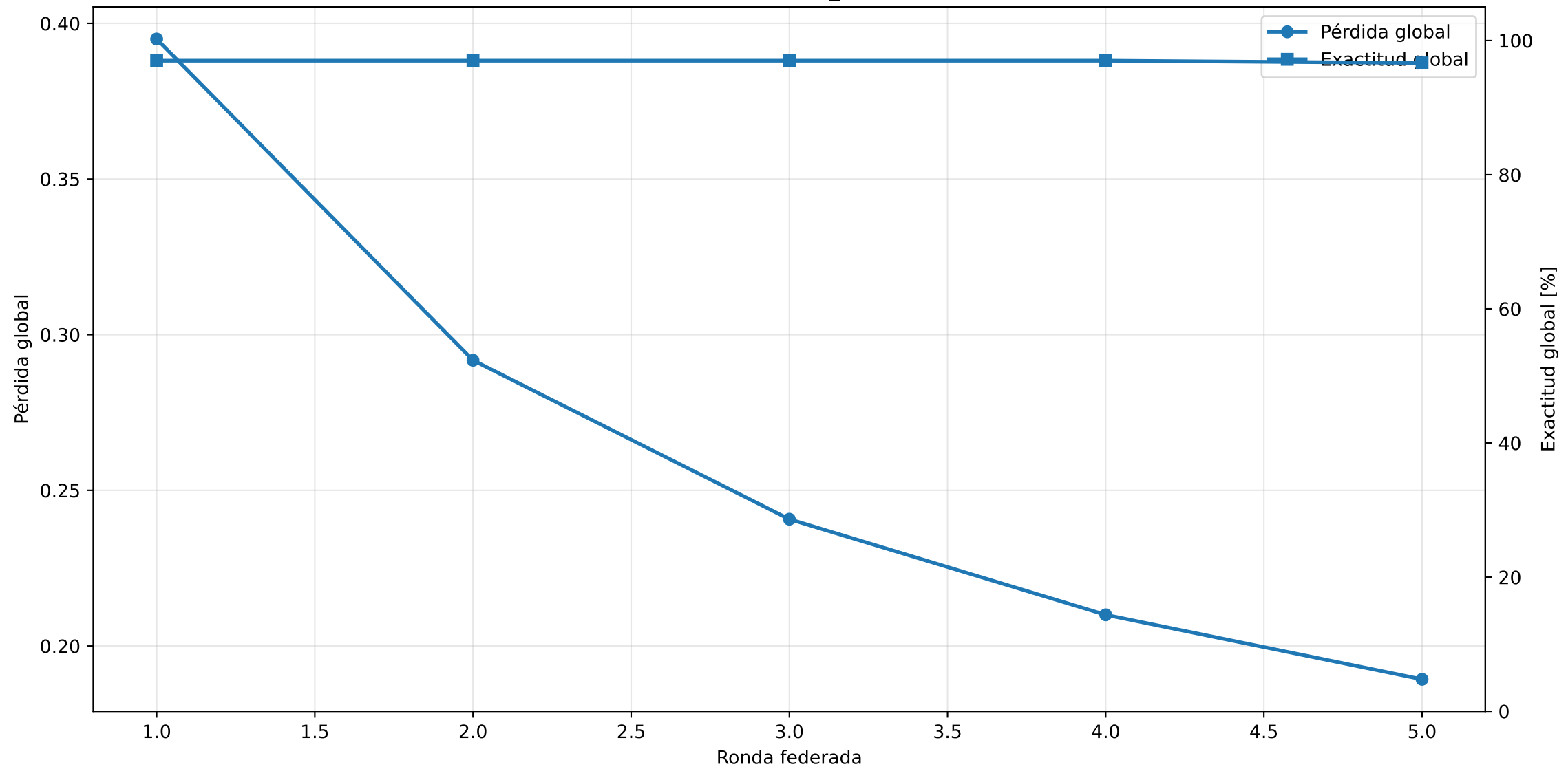
Aprendizaje federado FedAvg Escenario: LOW_POWER
