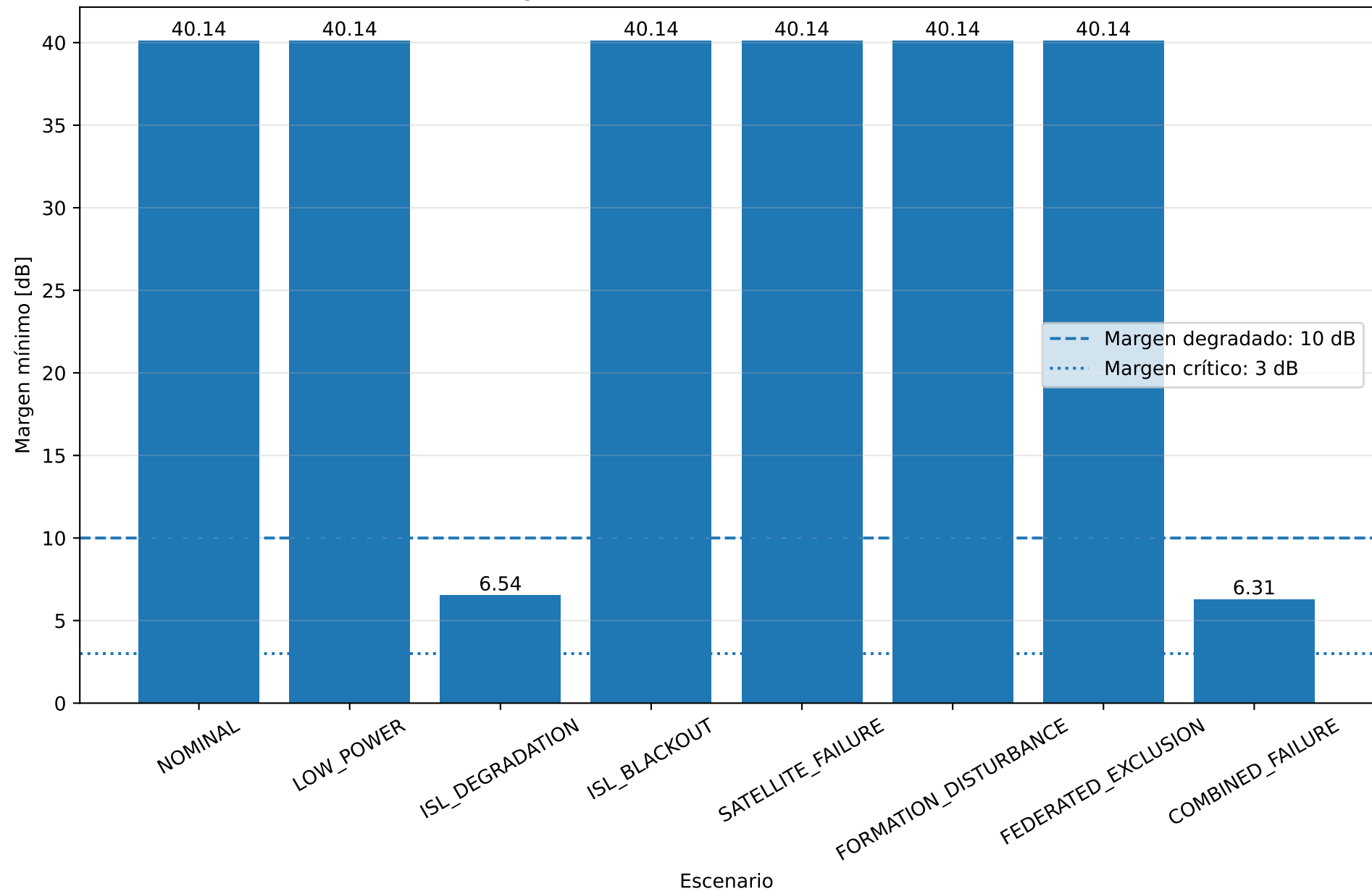
Margen mínimo del enlace intersatelital Ka
