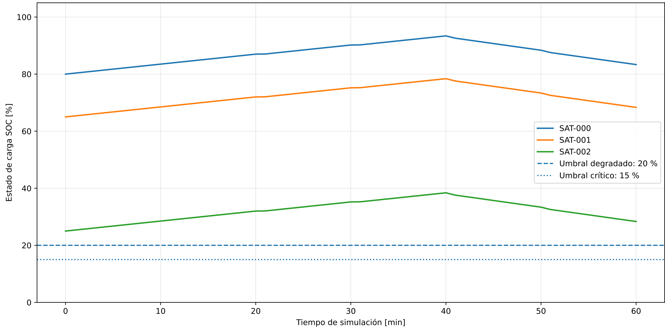
Evolución del estado de carga Escenario: NOMINAL
