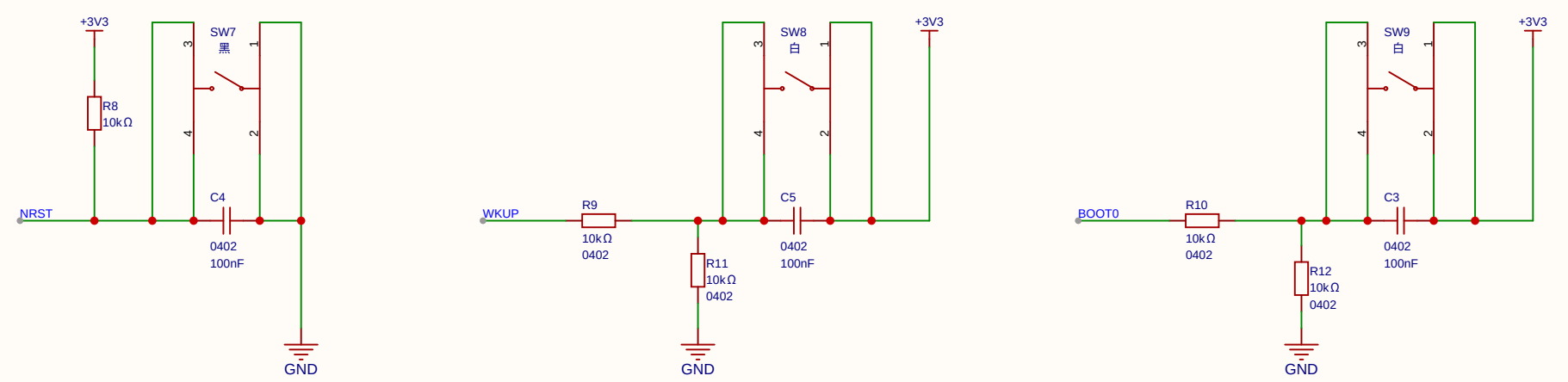
复位按键
