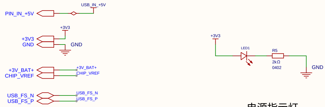
电源指示灯
