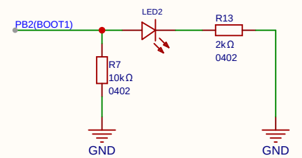
用户LED
