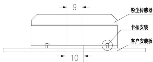
卡扣安装
