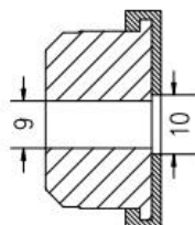
卡槽安装
