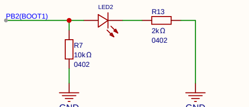
用户LED
