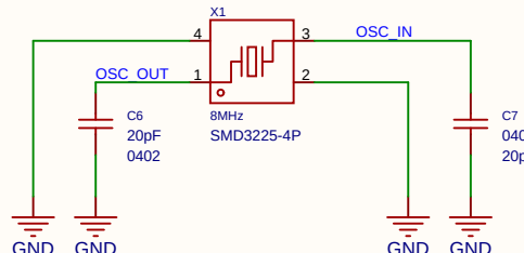
外部高速晶振
