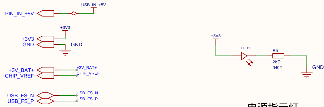
电源指示灯
