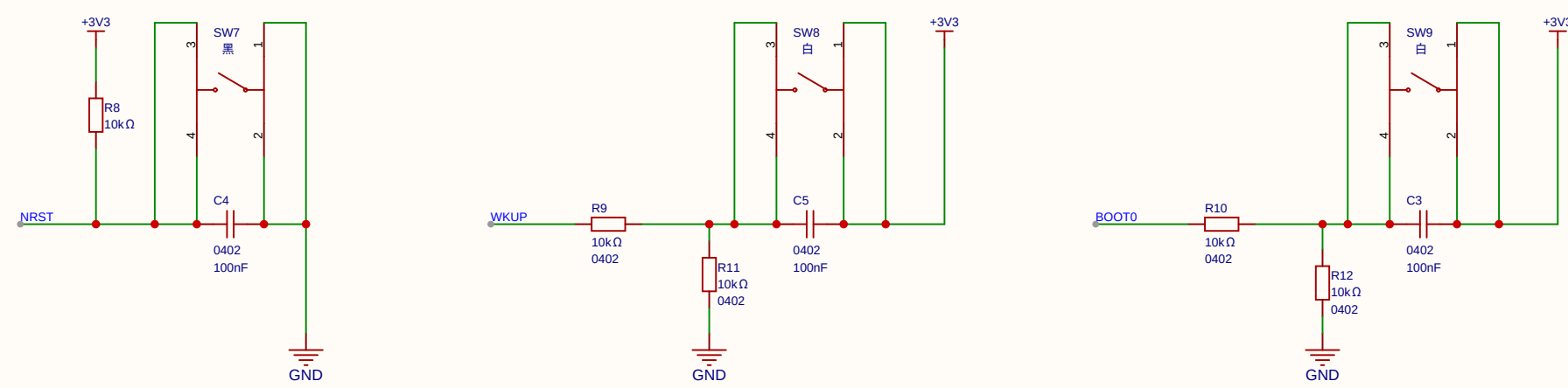
复位按键
