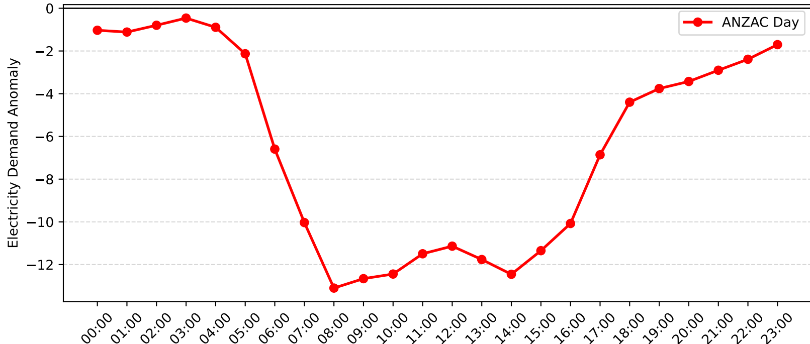
Zetland Demand Anomaly: ANZAC Day (2005-2006)
