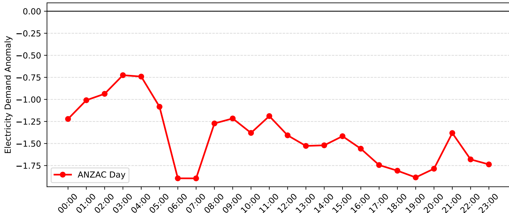
Morisset Demand Anomaly: ANZAC Day (2015-2016)
