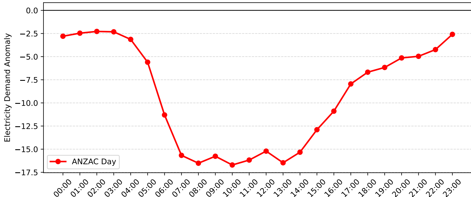
Milperra Demand Anomaly: ANZAC Day (2005-2006)
