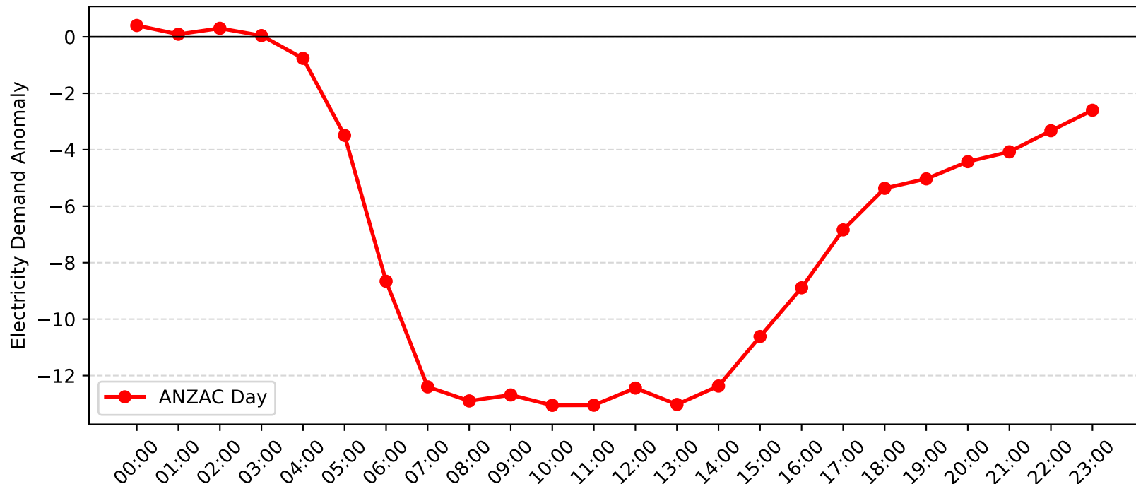
Milperra Demand Anomaly: ANZAC Day (2012-2013)
