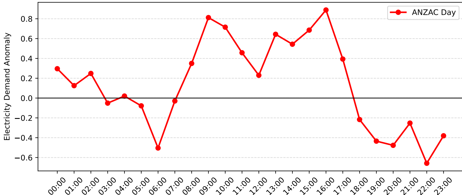
Swansea Demand Anomaly: ANZAC Day (2017-2018)
