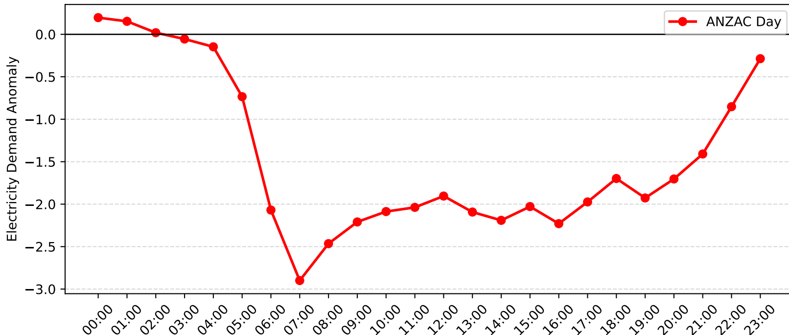
Rockdale Demand Anomaly: ANZAC Day (2009-2010)
