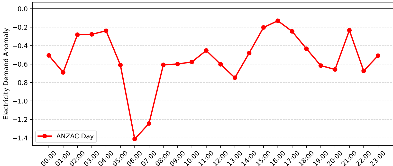
Morisset Demand Anomaly: ANZAC Day (2016-2017)
