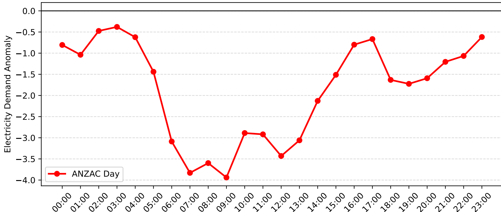
Wyong Demand Anomaly: ANZAC Day (2017-2018)
