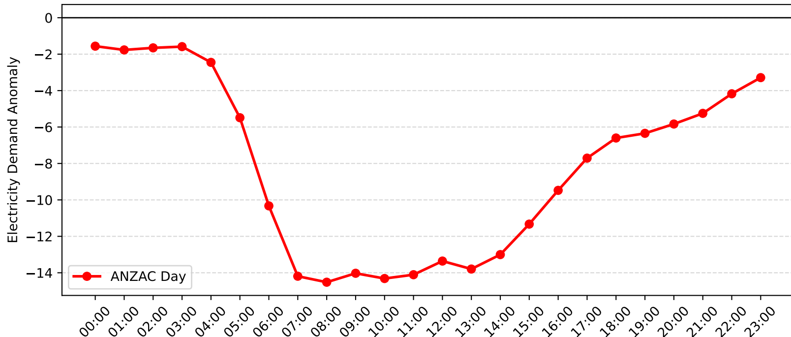
Milperra Demand Anomaly: ANZAC Day (2011-2012)
