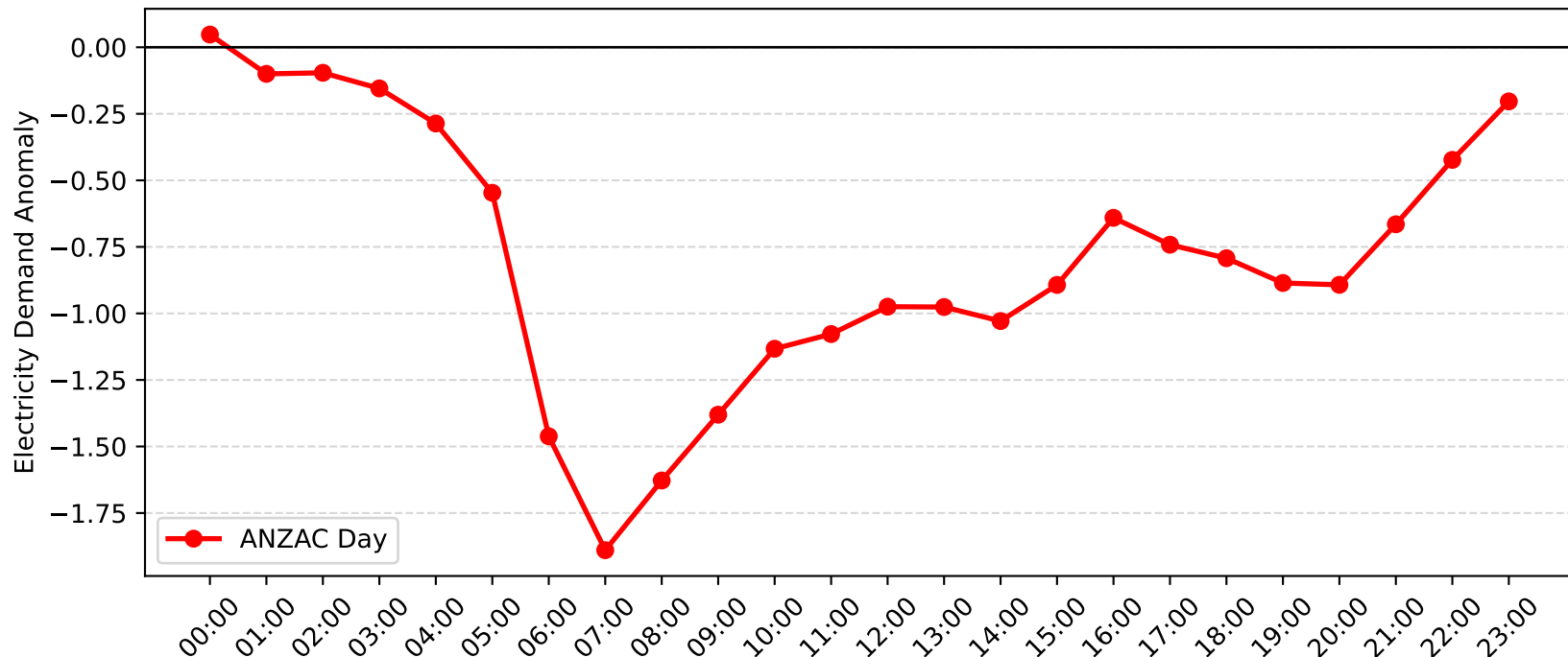
Rockdale Demand Anomaly: ANZAC Day (2015-2016)
