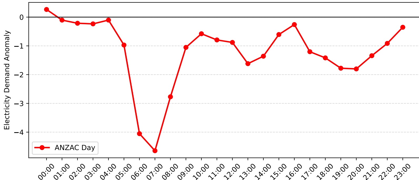
Mortdale Demand Anomaly: ANZAC Day (2015-2016)
