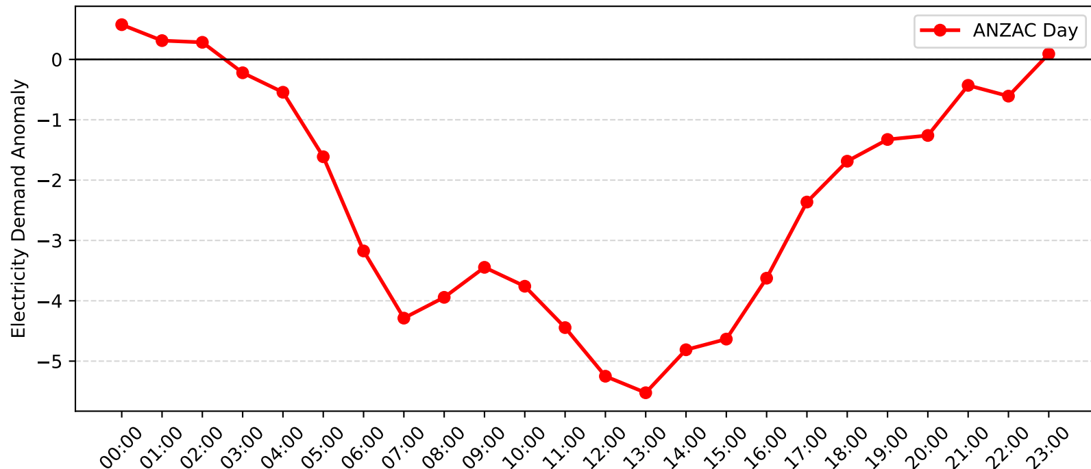
Wyong Demand Anomaly: ANZAC Day (2012-2013)
