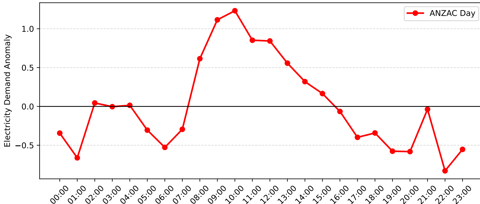
Swansea Demand Anomaly: ANZAC Day (2009-2010)
