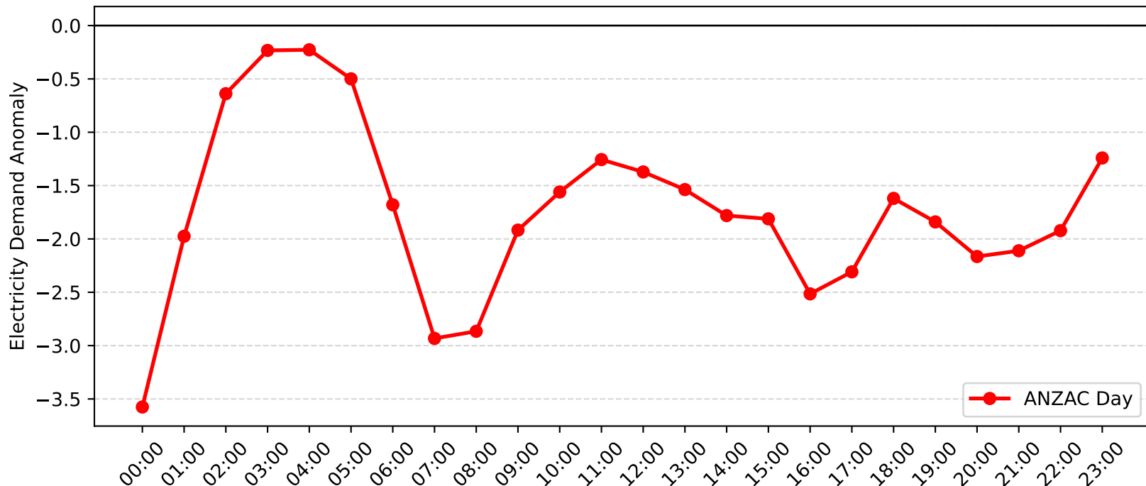
Mortdale Demand Anomaly: ANZAC Day (2004-2005)
