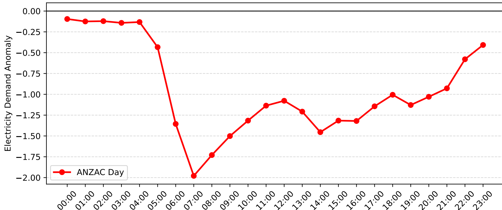
Rockdale Demand Anomaly: ANZAC Day (2013-2014)
