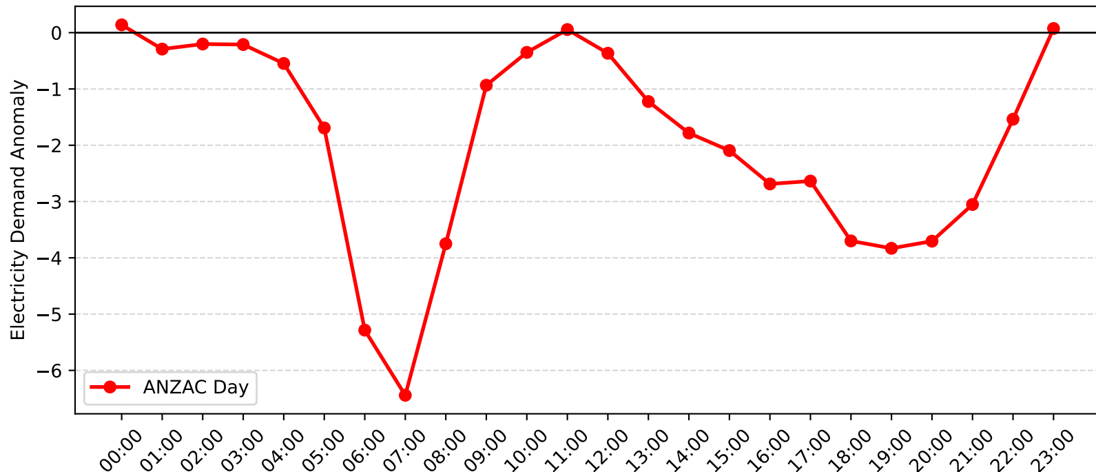
Mortdale Demand Anomaly: ANZAC Day (2008-2009)
