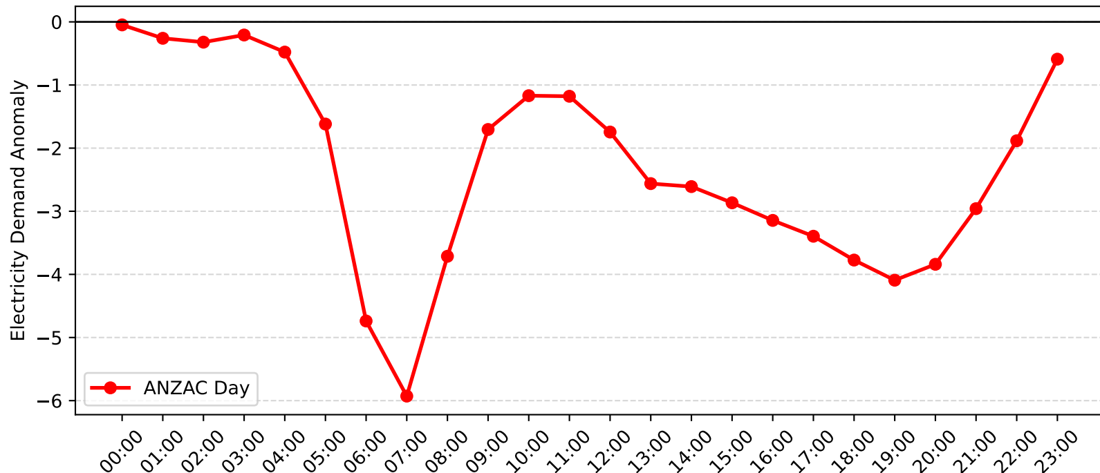
Mortdale Demand Anomaly: ANZAC Day (2009-2010)
