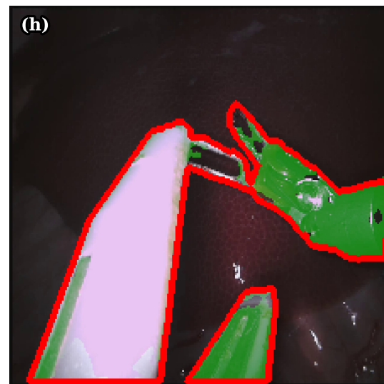
Prediction (Dice=0.909)
