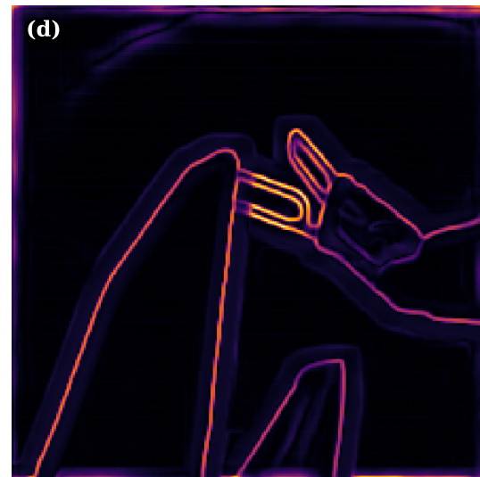
Prediction (Dice=0.909)
