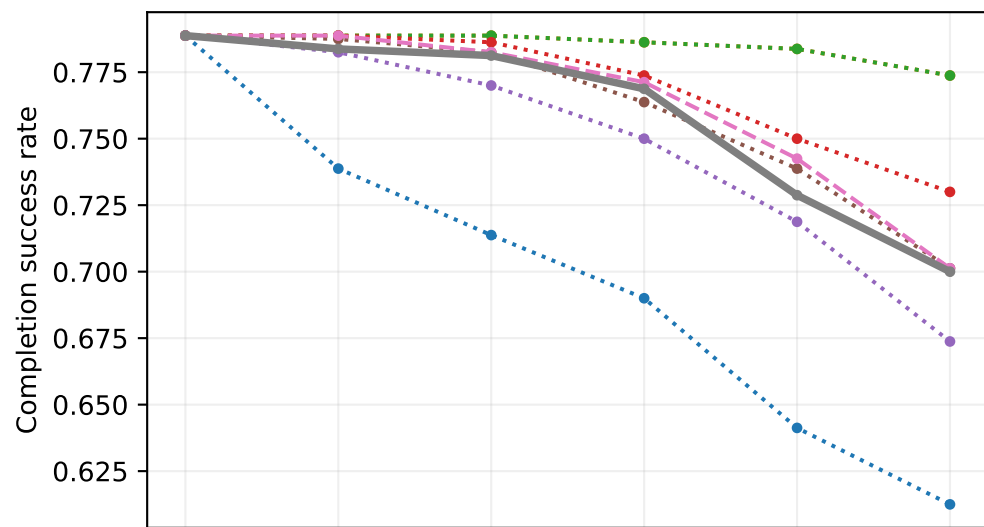
D* Lite
