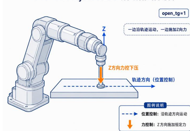
ForcePositionHybridControl 力位混合控制示意图
