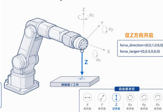
ForcePositionHybridControl 单轴力控示意图 (Z方向)
