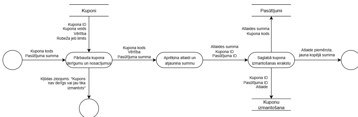
13. att. Kuponu pielietošanas datu plūsmas diagramma
