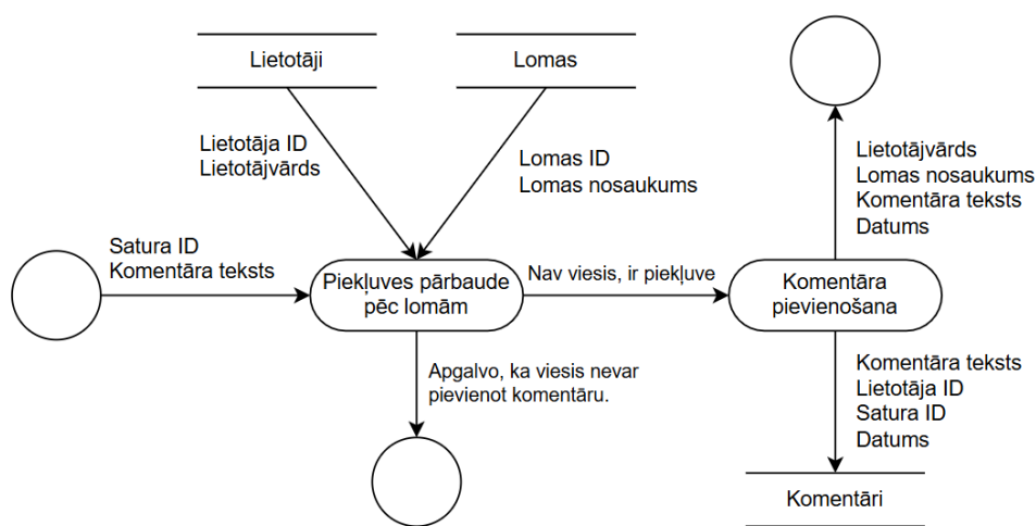
7. att. Komentāra pievienošanas datu plūsmu diagramma
