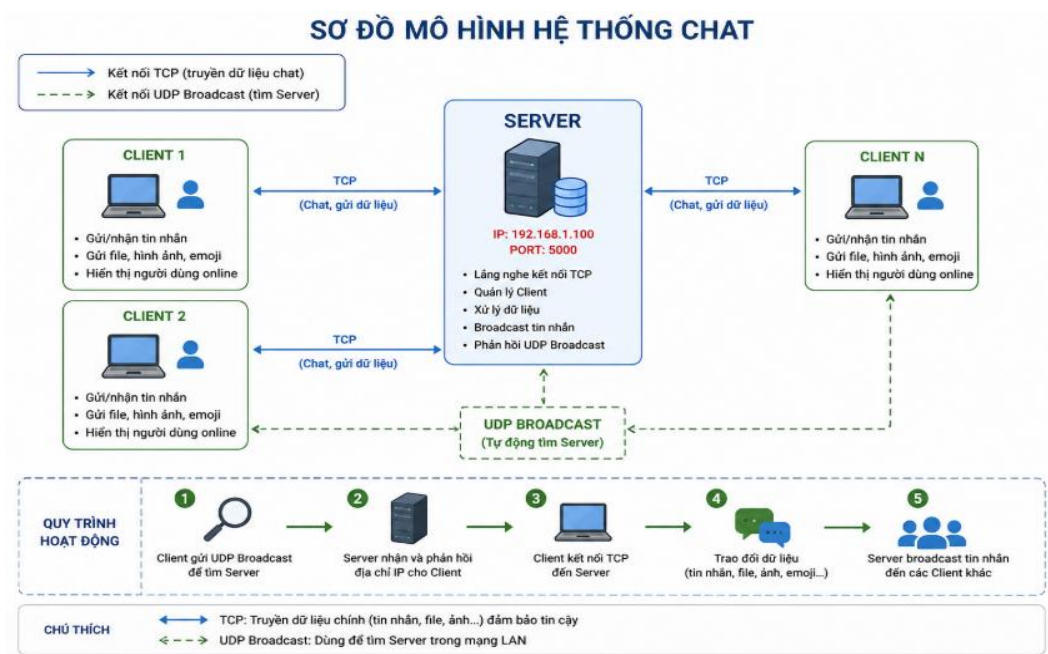
Hình 4.1: Sơ đồ hoạt động của hệ thống chat
