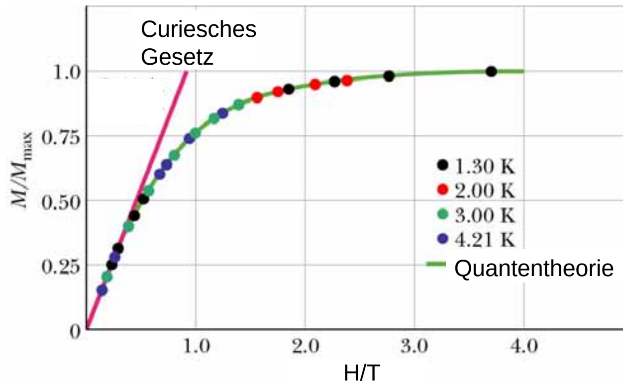
Magnetisierungskurve von Kaliumchromsulfat
