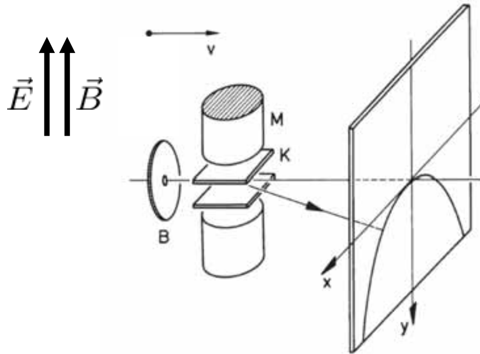
Parabelmethode zur Bestimmung der spezifischen Ladung
