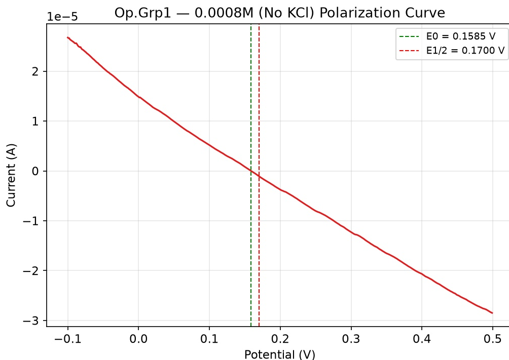
图 4: 0.0008M 无 KCl 极化曲线及半波电位
