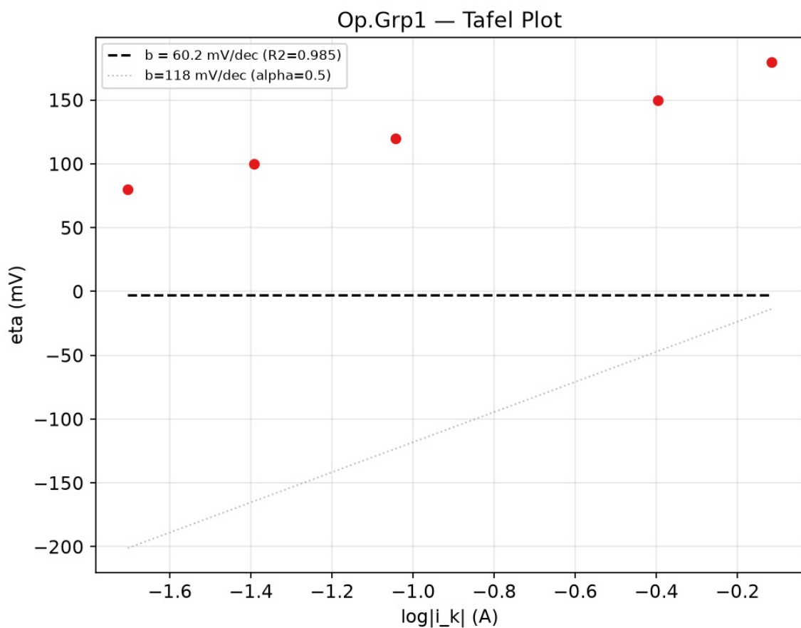
图 3: Tafel 图 (Grp1): \eta vs \log|i_k| 。虚线为 b = 118 mV/dec ( \alpha = 0.5 ) 参考线。
