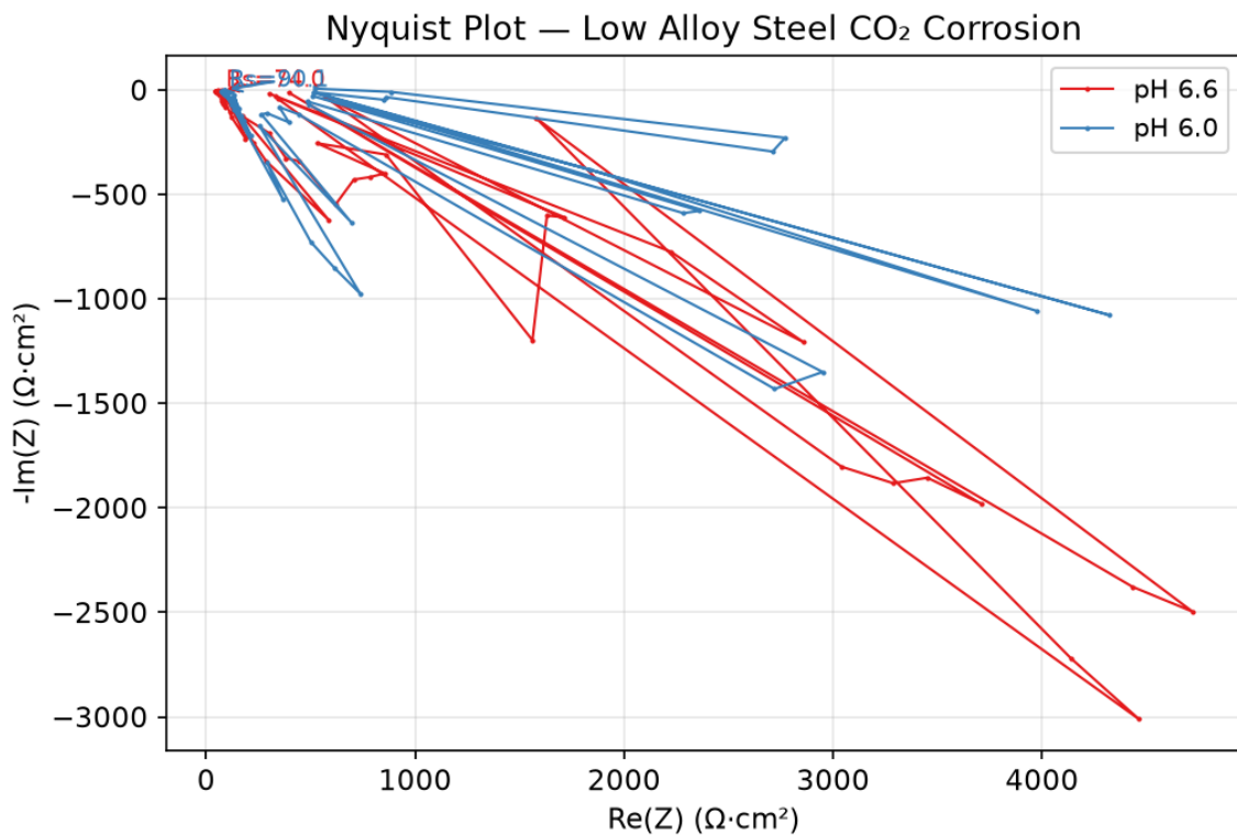
图 1: Nyquist 图: pH 6.0 vs 6.6 对比。两个体系均呈现单一严重压扁的容抗弧 ( n < 0.6 ), 表明腐蚀产物层表面高度不均匀。pH 6.6 的弧直径显著更大, 反映更高的极化电阻。
