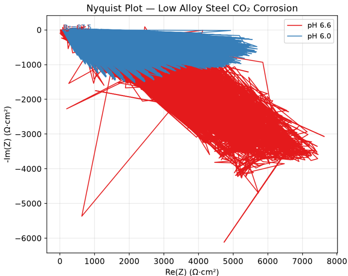
图 1: Nyquist 图: pH 6.0 vs 6.6 对比。两个体系均呈现单一严重压扁的容抗弧 ( n < 0.6 ), 表明腐蚀产物层表面高度不均匀。pH 6.6 的弧直径显著更大, 反映更高的极化电阻。
