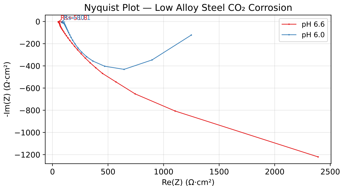
图 1: Nyquist 图: pH 6.0 vs 6.6 对比。两个体系均呈现单一严重压扁的容抗弧 ( n < 0.6 ), 表明腐蚀产物层表面高度不均匀。pH 6.6 的弧直径显著更大, 反映更高的极化电阻。
