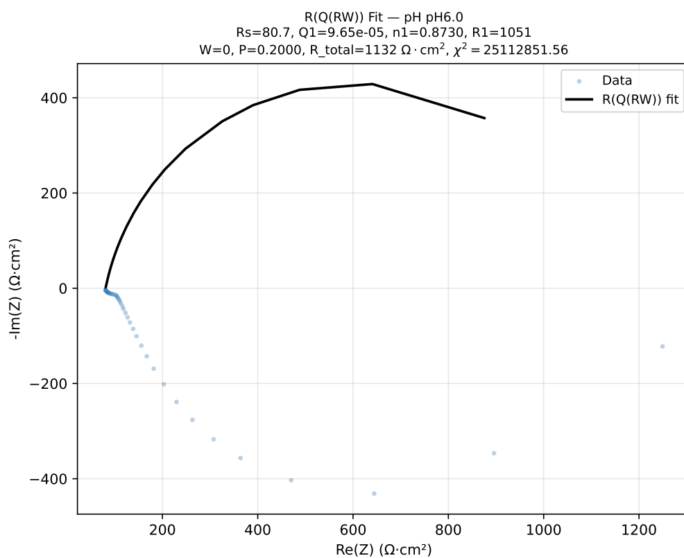
图 4: pH 6.0 —R(Q(RW)) 拟合 Nyquist 图
