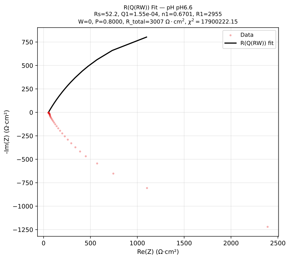
图 3: pH 6.6 —R(Q(RW)) 拟合 Nyquist 图
