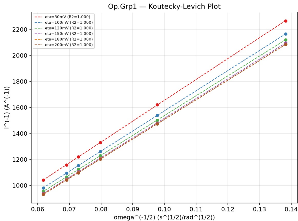
图 3: K-L 图 (Grp1): 1/|i| vs \omega^{-1/2} , 6 个过电位各一条拟合线
