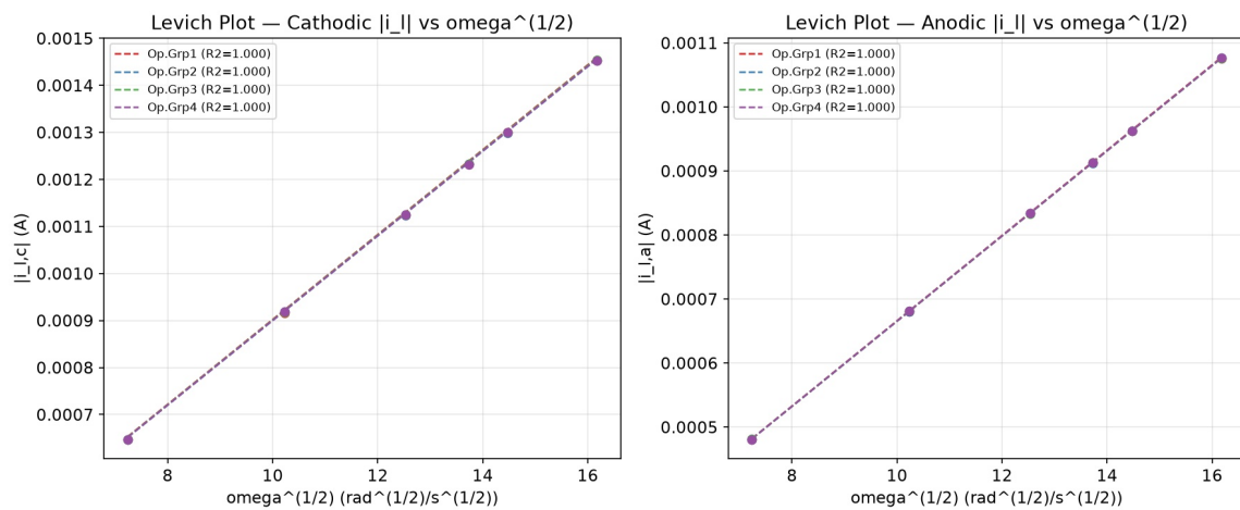
图 1: Levich 图: 阴极 |i_l| vs \omega^{1/2} (左) 与阳极 |i_l| vs \omega^{1/2} (右)。4 条线几乎重合, 反映 4 组独立测量的高度一致性。
