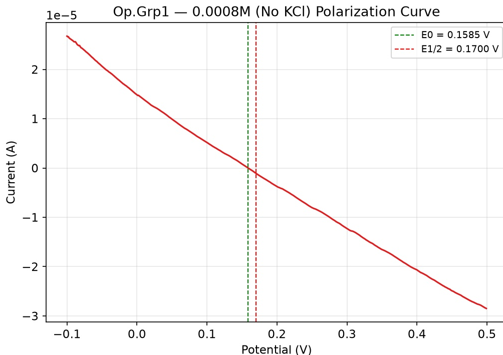
图 5: 0.0008M 无 KCl 极化曲线及半波电位
