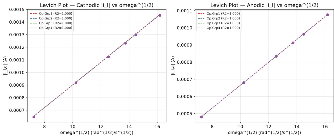
图 2: Levich 图: 阴极 |i_l| vs \omega^{1/2} (左) 与阳极 |i_l| vs \omega^{1/2} (右)。4 条线几乎重合, 反映 4 组独立测量的高度一致性。
