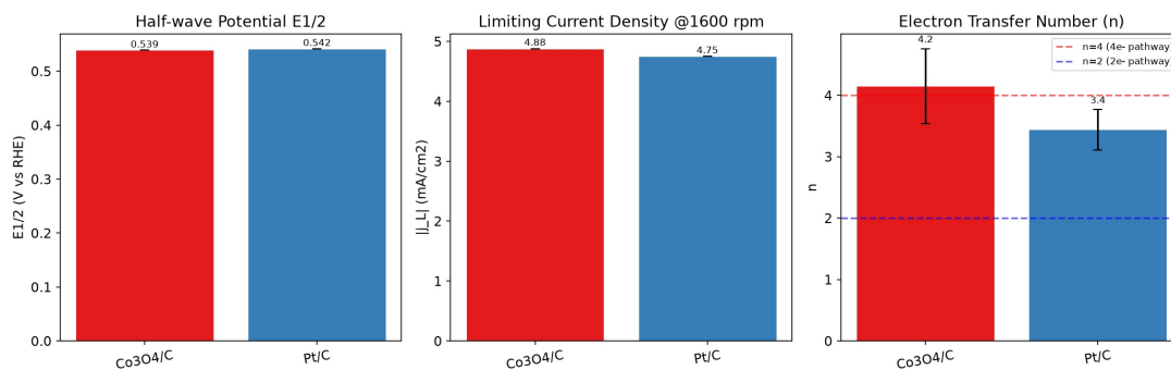
图 4: 关键电化学参数对比: 半波电位 E_{1/2} 、极限电流密度 |j_L| 、电子转移数 n
