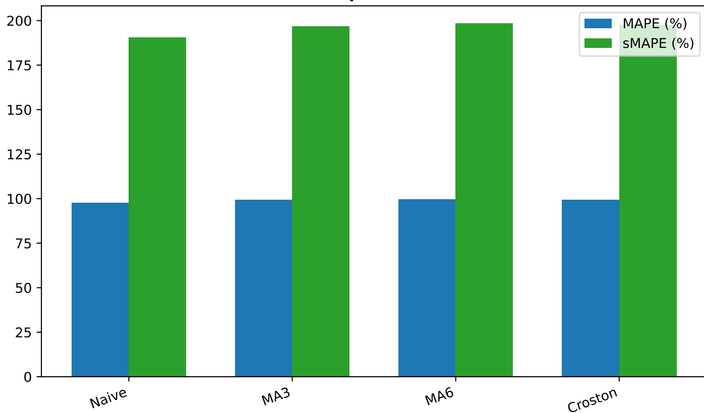
Sai số Tương đối - Mã: 47.L1.6060.AFP9660(0,4,7) (Vô địch: Naive)
