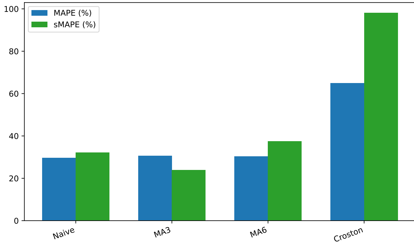
Sai số Tương đối - Mã: 29.L1.3060.FUSM3647(D) (Vô địch: MA3)
