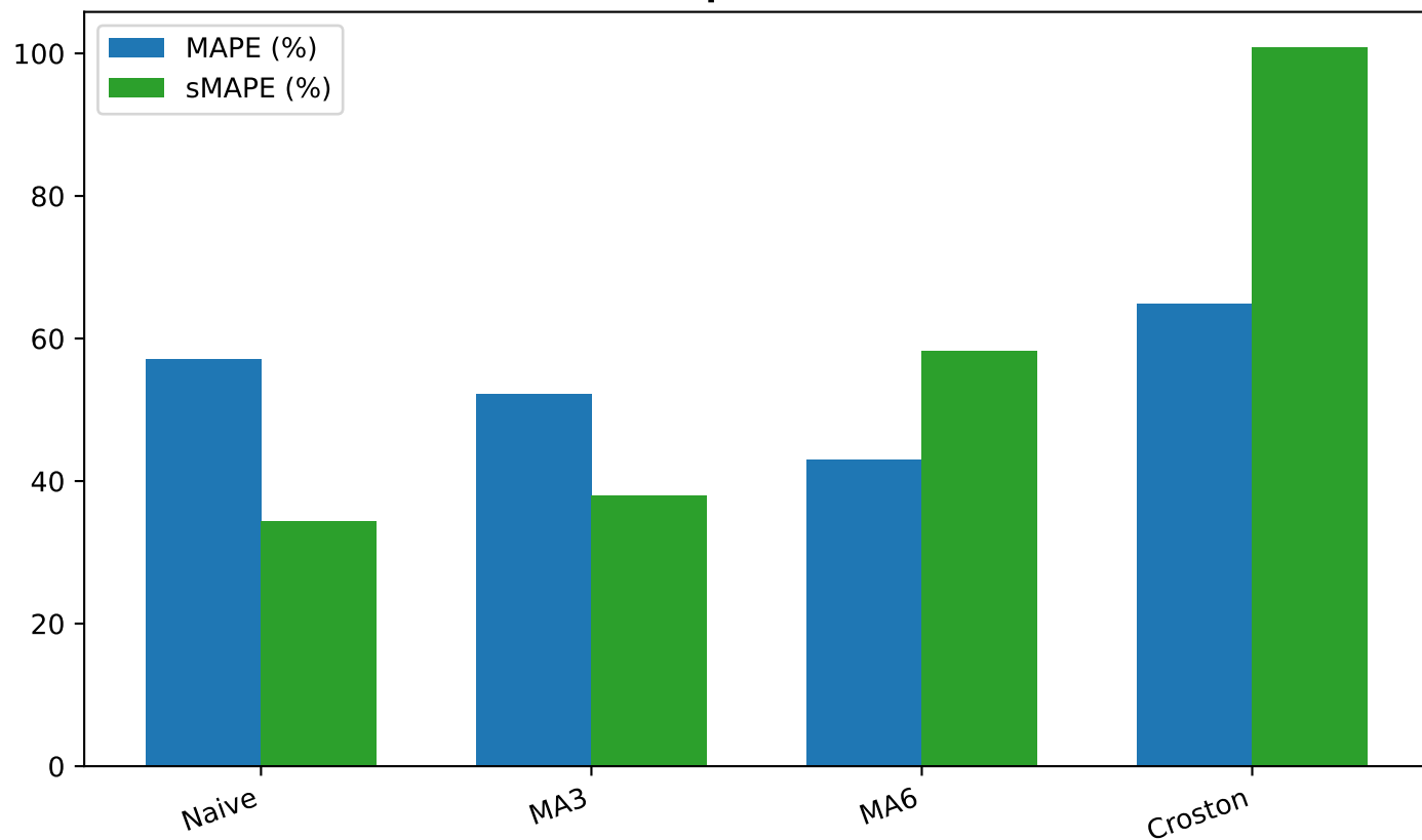
Sai số Tương đối - Mã: 20.L1.6060.A8960(1-7) (Vô địch: Naive)
