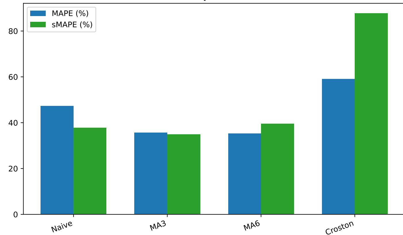
Sai số Tương đối - Mã: 29.L1.3060.FUSC3636 (Vô địch: MA3)
