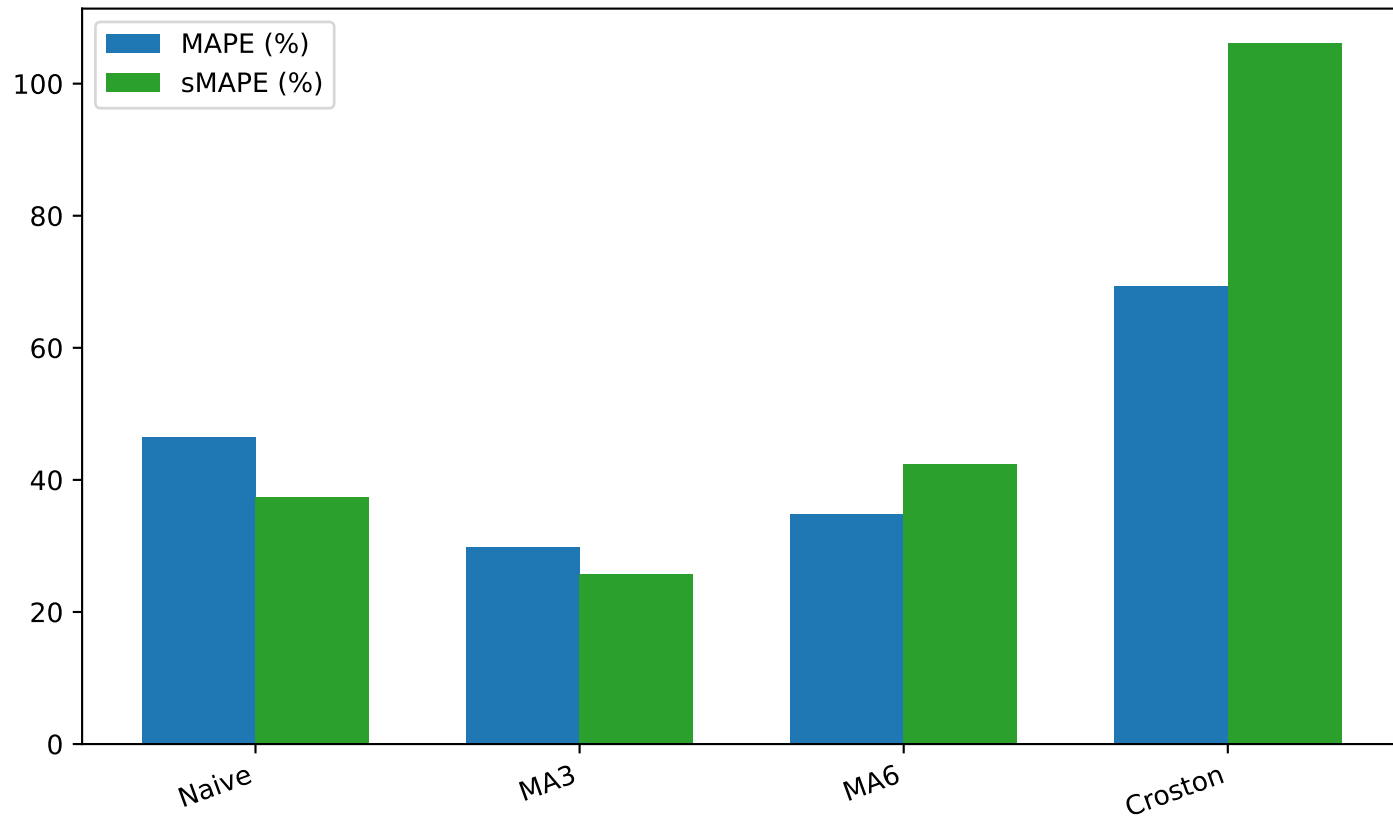
Sai số Tương đối - Mã: 25.L1.4080.FP948603(D,V) (Vô địch: MA3)
