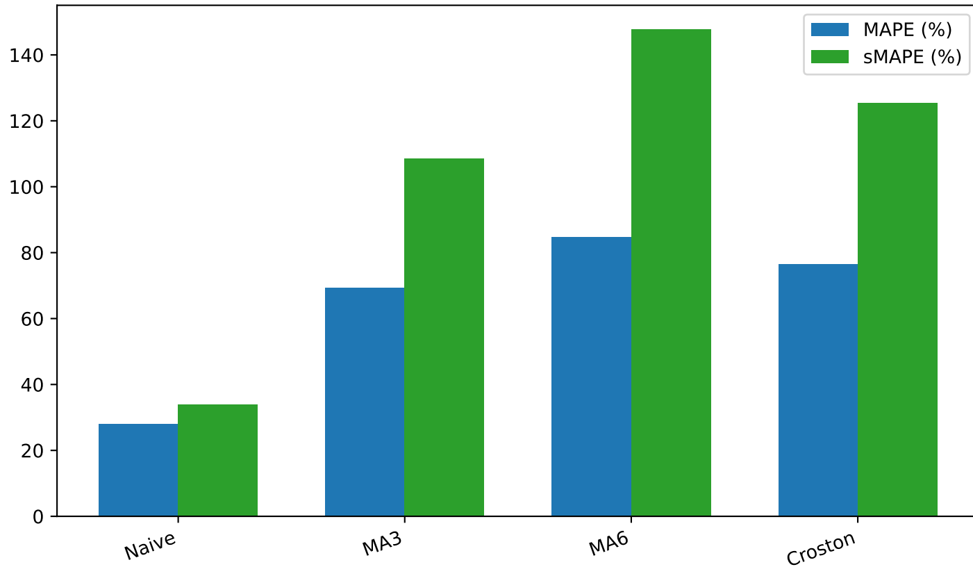
Sai số Tương đối - Mã: 38.L1.4080.UT481002(D,V) (Vô địch: Naive)
