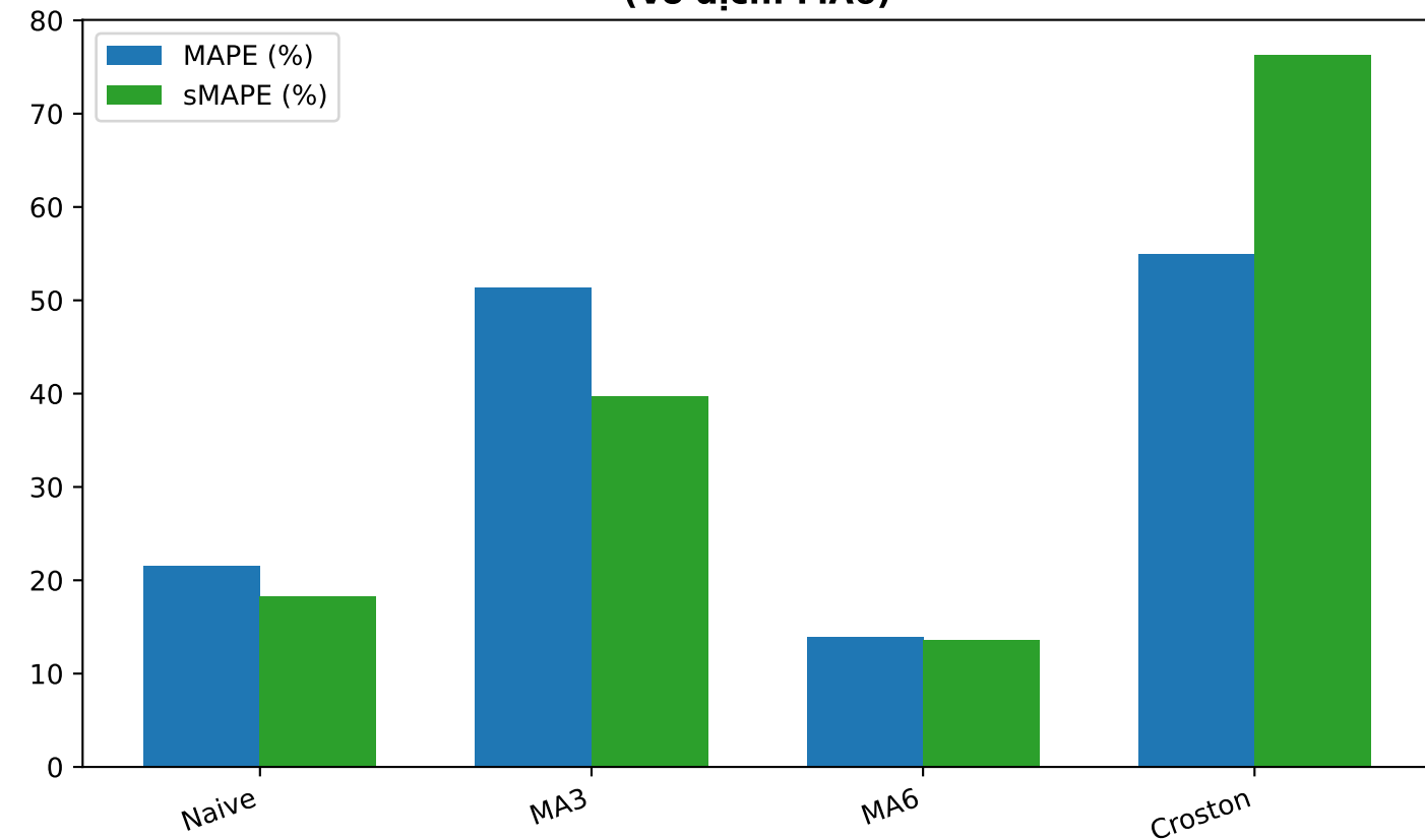
Sai số Tương đối - Mã: 20.L1.6060.A16(114,405) (Vô địch: MA6)
