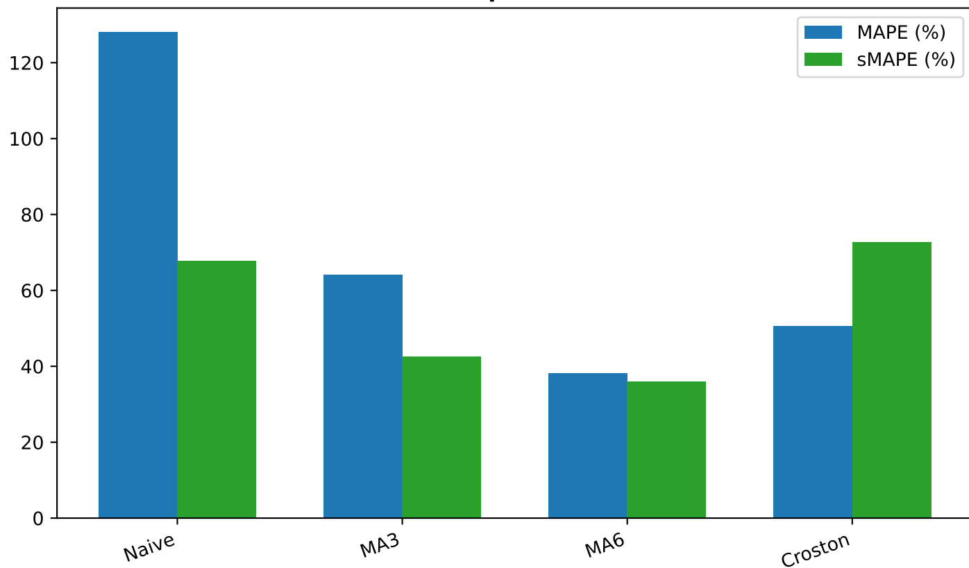
Sai số Tương đối - Mã: 25.L1.3060.FP936605 (Vô địch: MA6)
