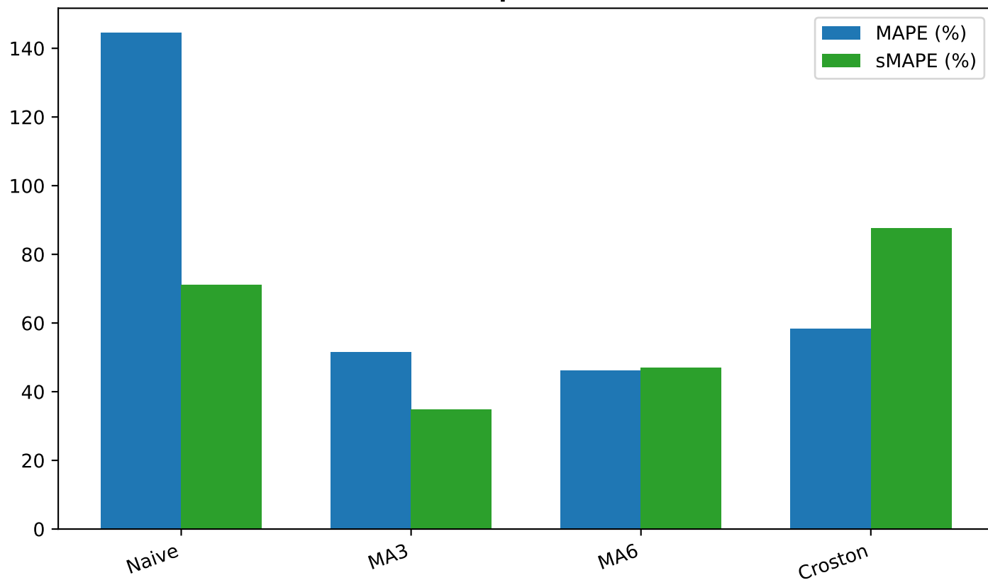
Sai số Tương đối - Mã: 25.L1.8080.FP1860(0,1,4,6,7,8) (Vô địch: MA3)
