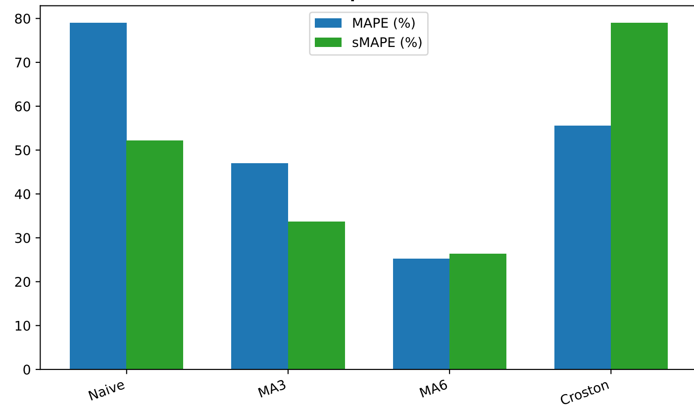
Sai số Tương đối - Mã: 29.L1.3060.FUSM3648 (Vô địch: MA6)
