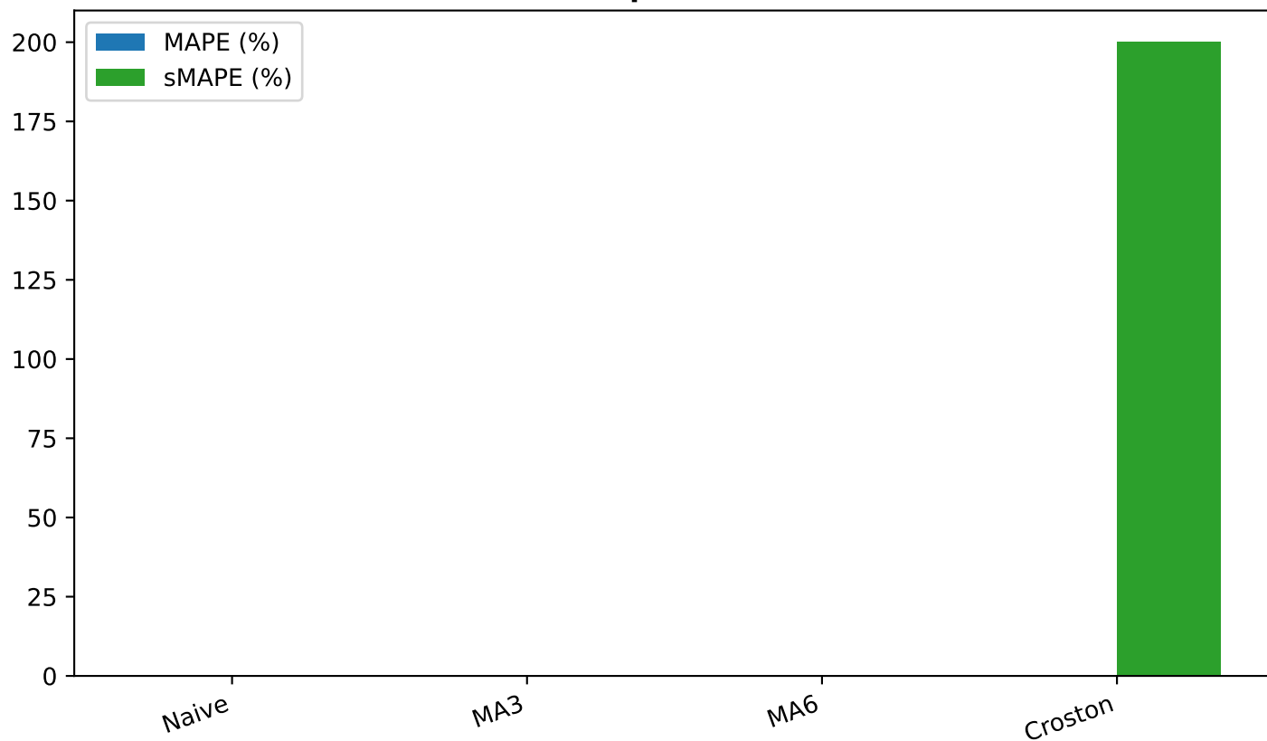
Sai số Tương đối - Mã: 00.L1.8080.P87625N (Vô địch: Naive)
