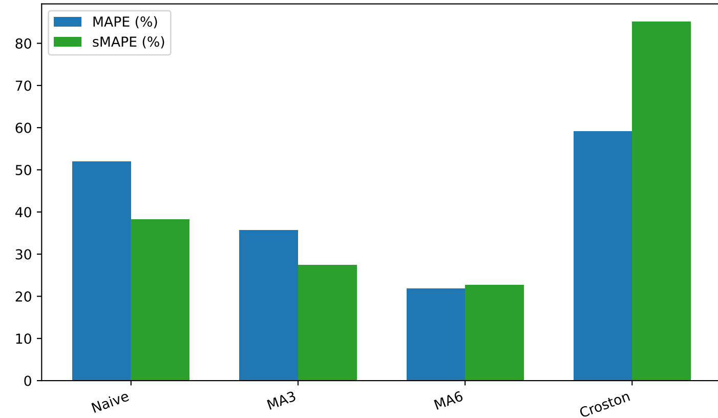
Sai số Tương đối - Mã: 20.L1.6060.A6610(1-6) (Vô địch: MA6)
