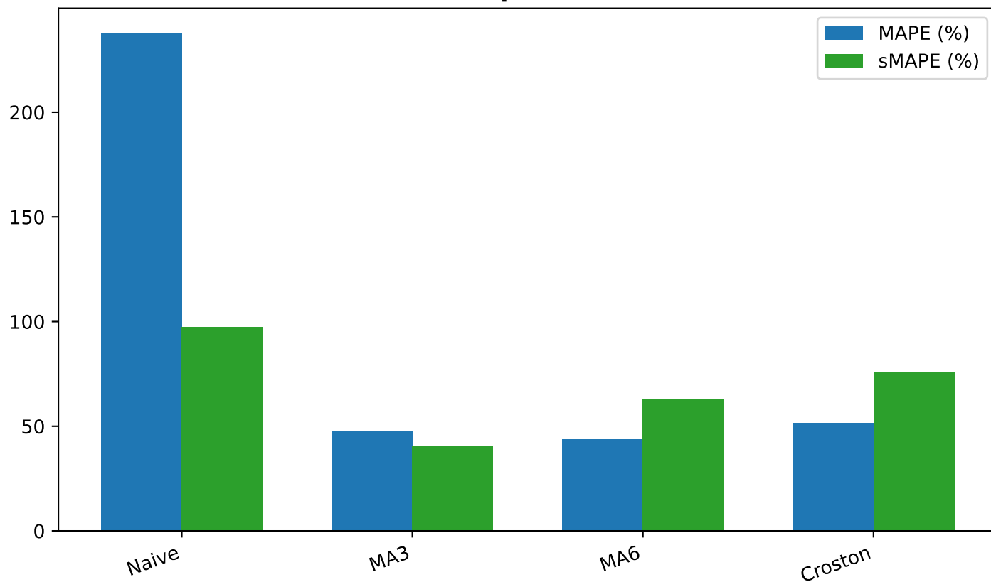
Sai số Tương đối - Mã: 41.L1.3060.MS36100(1T,2D,3V) (Vô địch: MA3)
