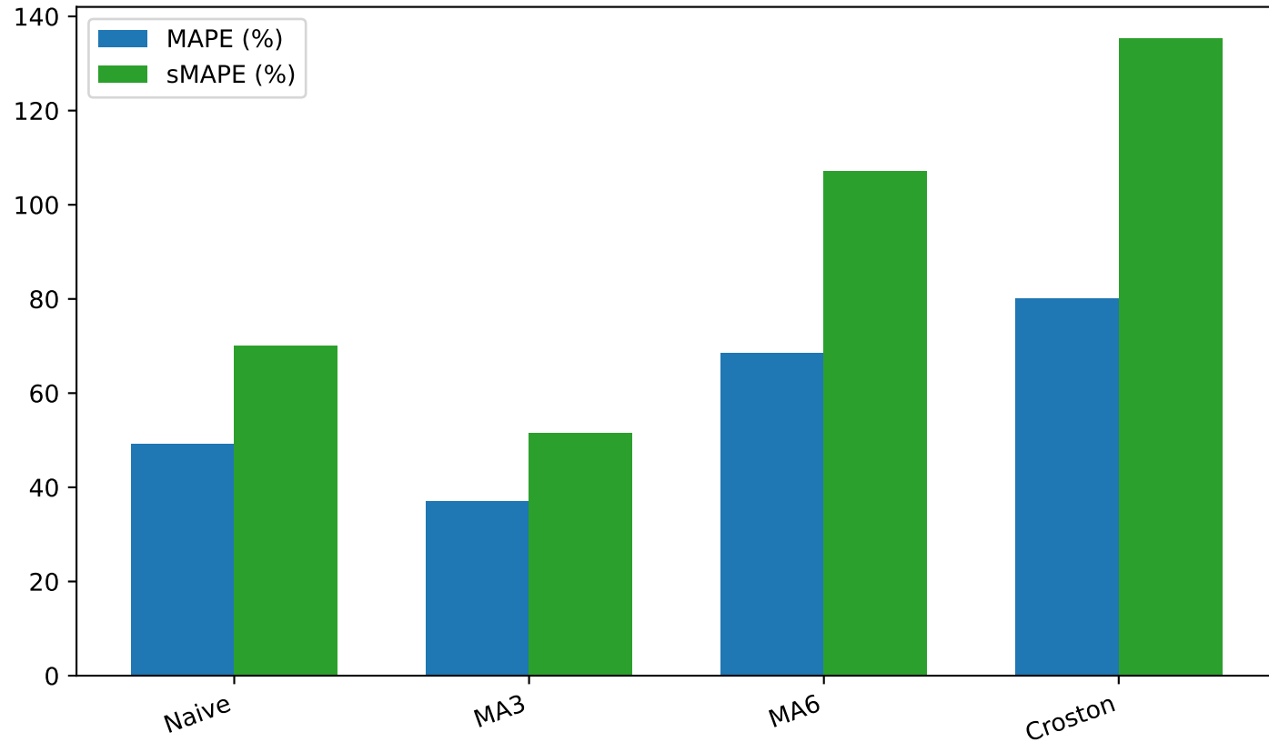
Sai số Tương đối - Mã: 05.L1.3060.KAG36905 (Vô địch: MA3)
