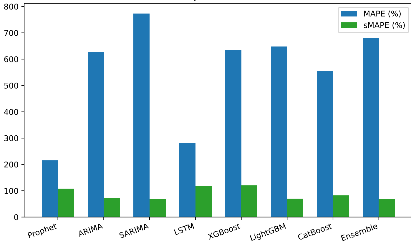
Sai số Tương đối - Mã: 22.C200.DG.TBOND.00 (Vô địch: Ensemble)
