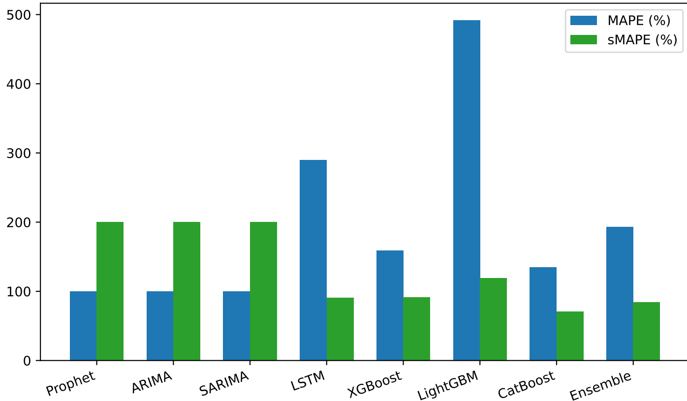
Sai số Tương đối - Mã: 14.L1.3060.US36CG80(2,4) (Vô địch: CatBoost)
