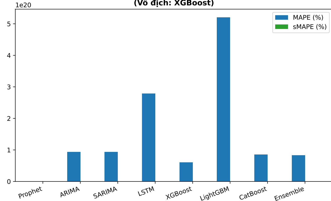
Sai số Tương đối - Mã: 10.L1.3060.579x (Vô địch: XGBoost)
