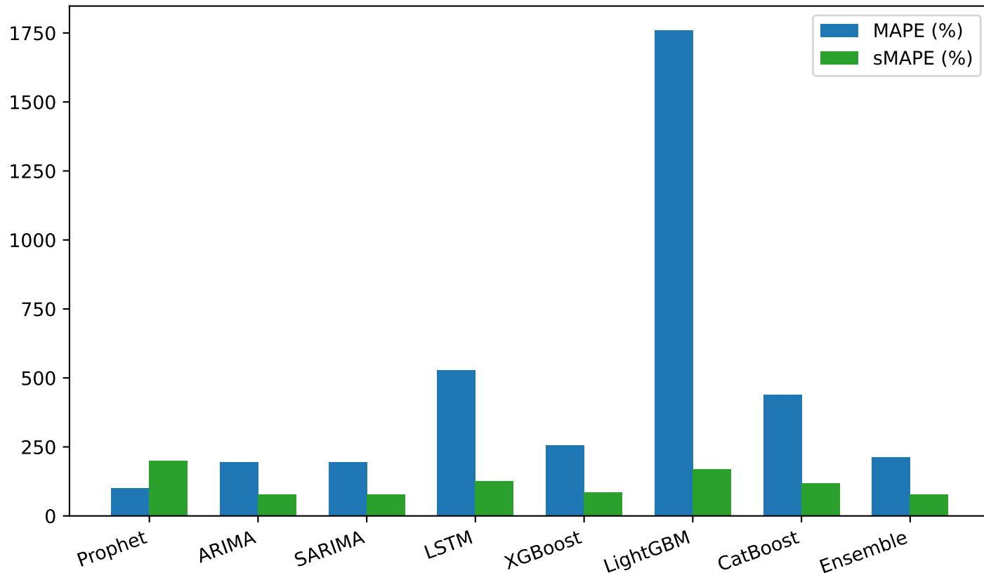
Sai số Tương đối - Mã: 14.L1.3030.333(16,18,20) (Vô địch: Ensemble)
