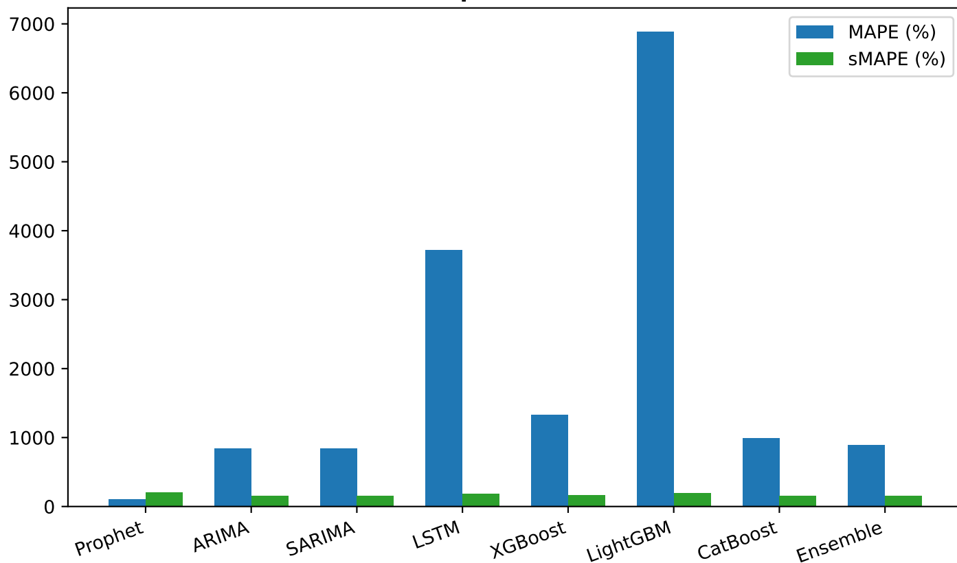
Sai số Tương đối - Mã: 12.L1.3030.302(0,1,2,3,4,6) (Vô địch: CatBoost)
