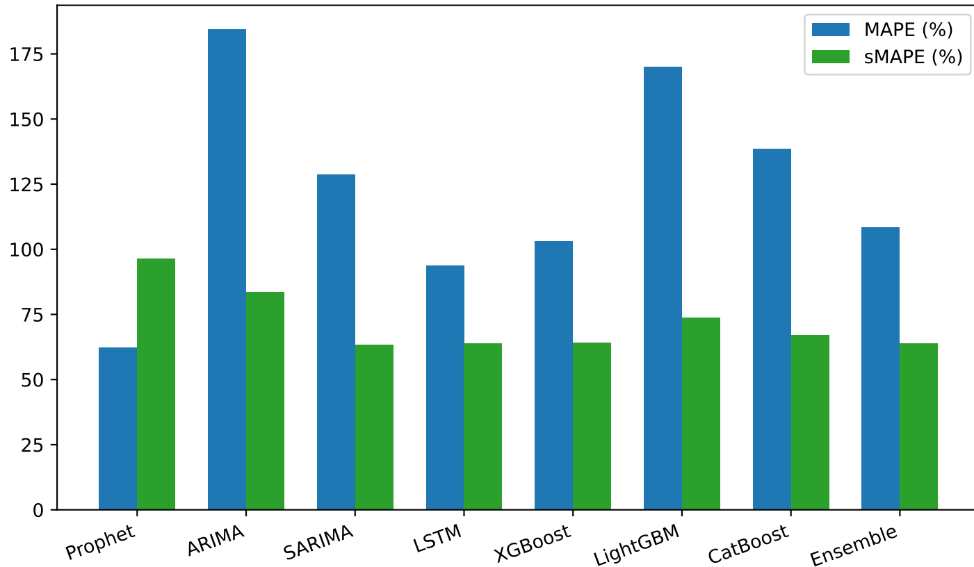
Sai số Tương đối - Mã: 20.L1.6060.86301 (Vô địch: SARIMA)
