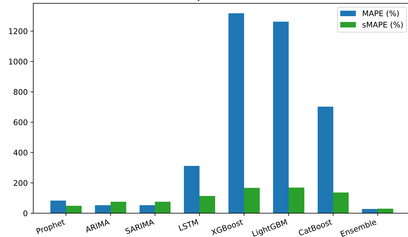
Sai số Tương đối - Mã: 15.L1.6060.660(1,2,4,5,6) (Vô địch: Ensemble)
