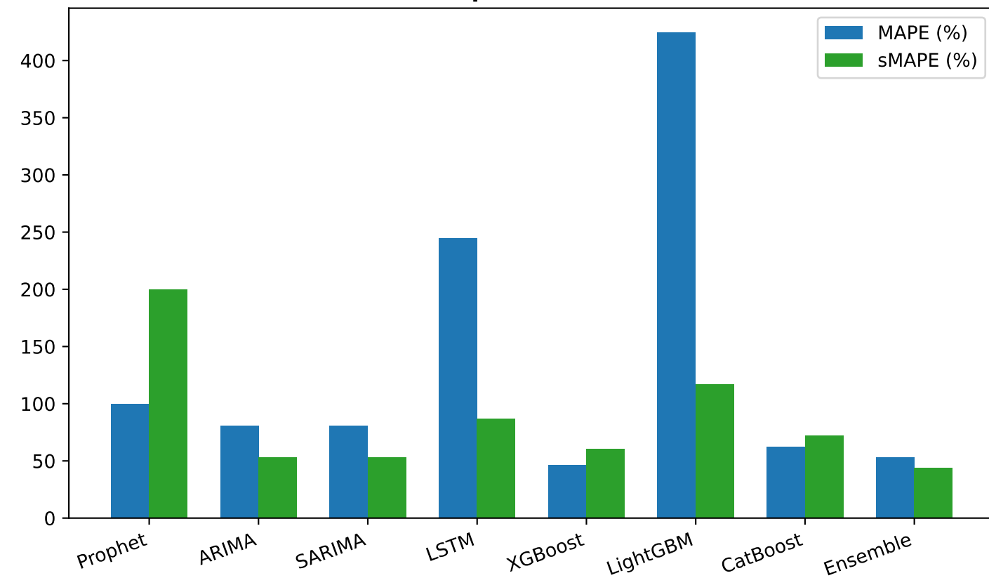
Sai số Tương đối - Mã: 29.L1.3060.FC3618(D) (Vô địch: Ensemble)
