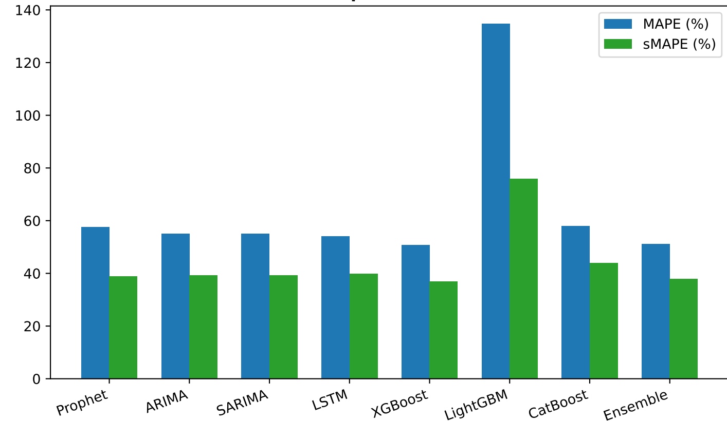
Sai số Tương đối - Mã: 14.L1.3060.A369(10,22) (Vô địch: XGBoost)
