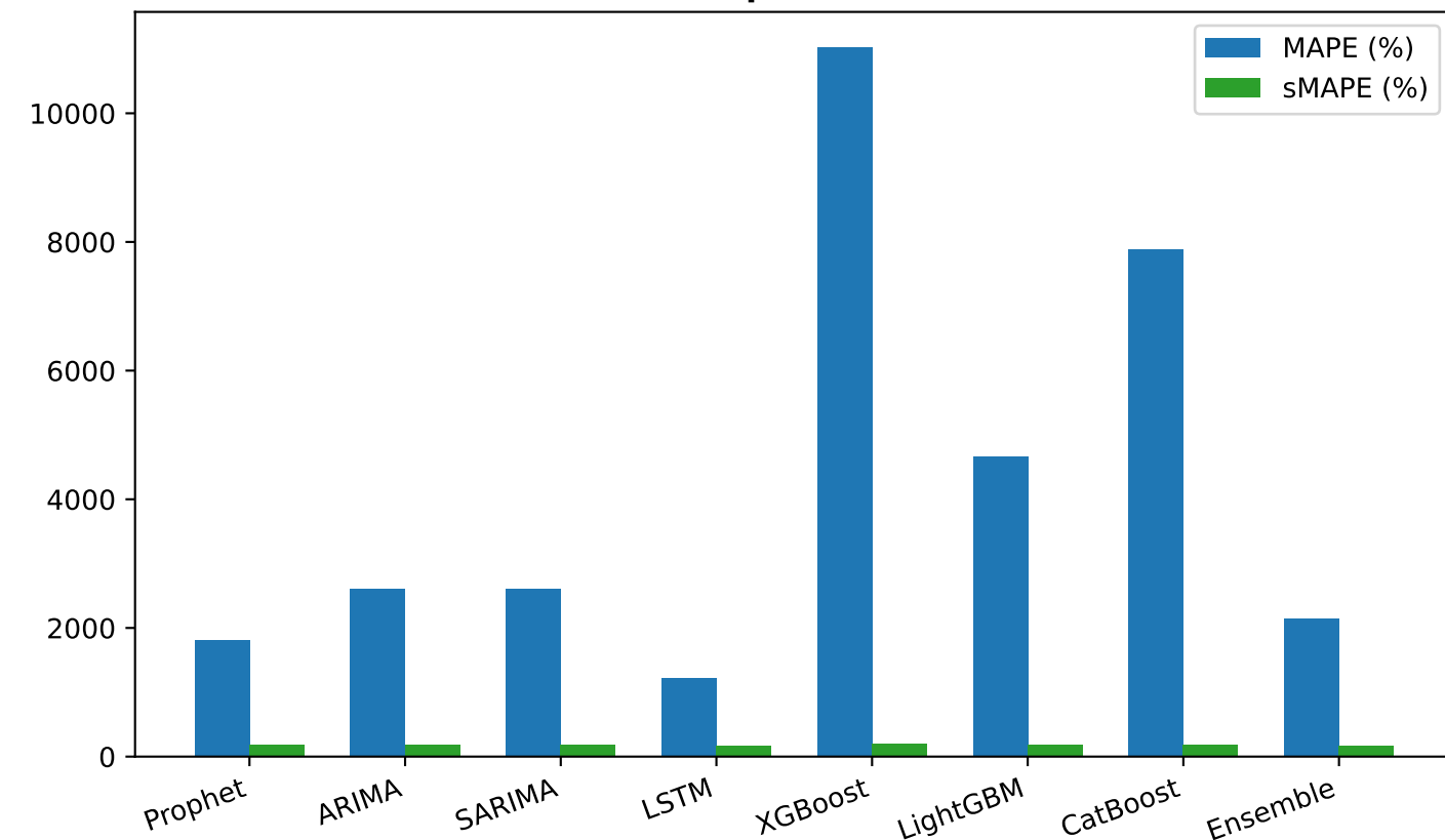
Sai số Tương đối - Mã: 10.L1.6060.615x-6x (Vô định: LSTM)
