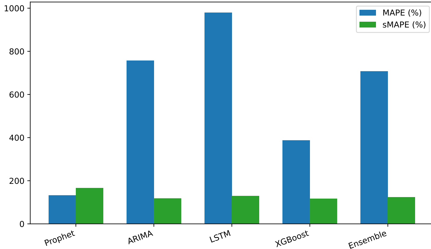
Sai số Tương đối - Mã: 14.L1.4080.488(00,07,68) (Vô địch: XGBoost)
