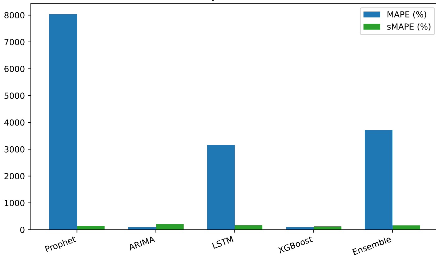
Sai số Tương đối - Mã: 09.L1.1590.CA09GK1590X (Vô địch: XGBoost)
