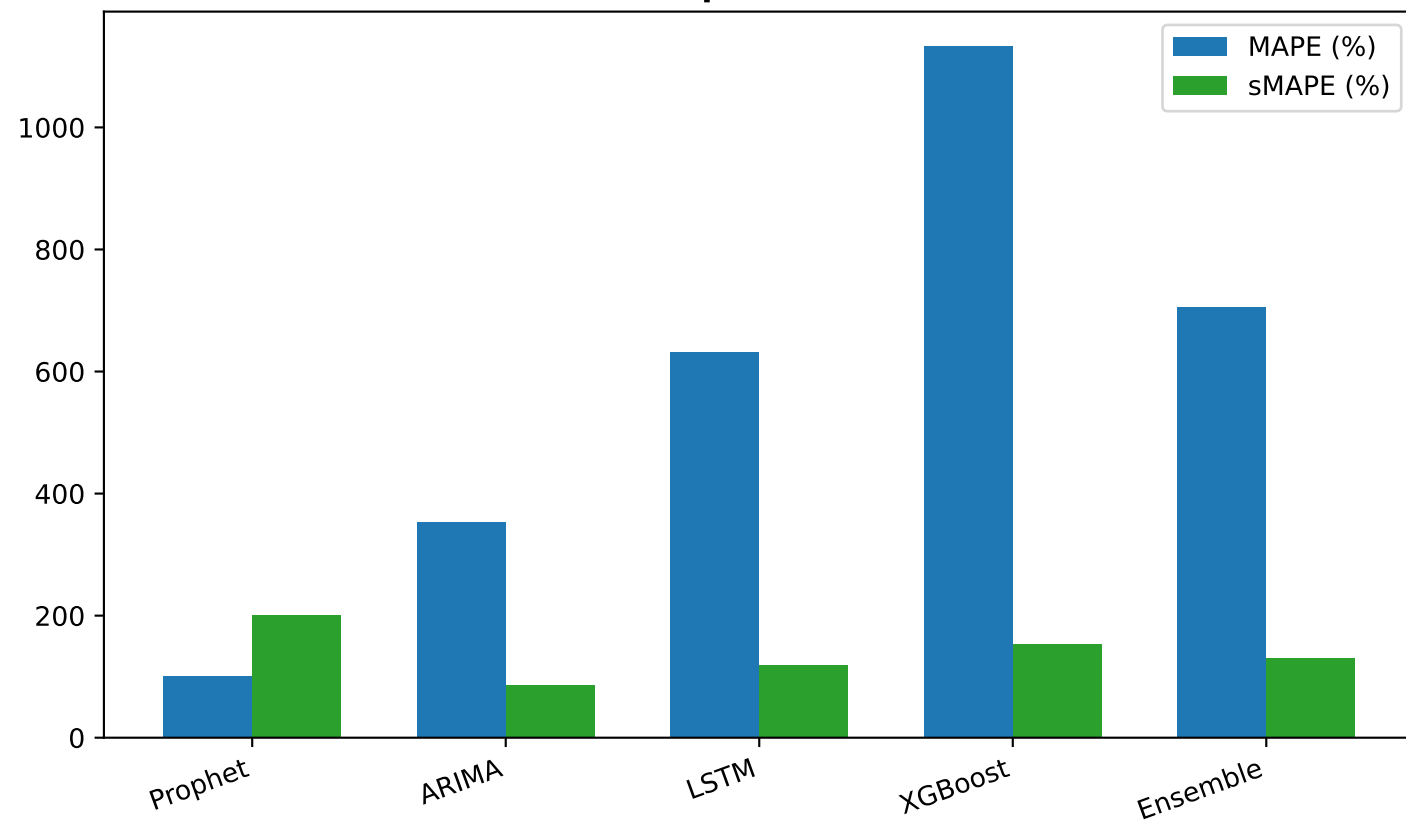
Sai số Tương đối - Mã: 14.L1.3060.US36CB(806,902/902D) (Vô địch: ARIMA)
