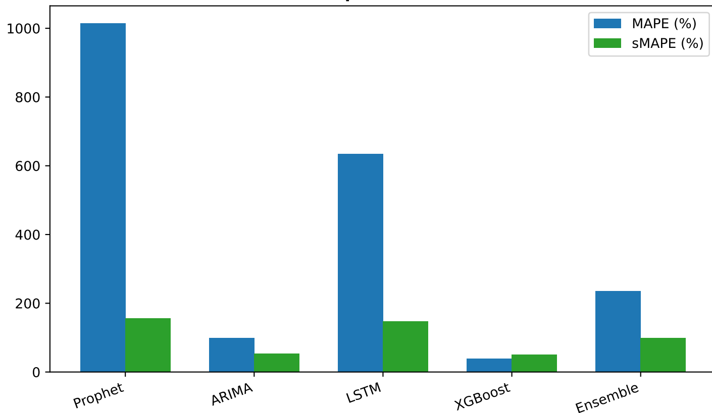
Sai số Tương đối - Mã: 34.L1.ITA-060120-00x (Vô địch: XGBoost)
