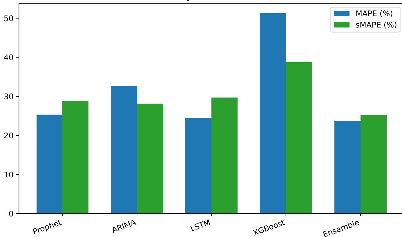
Sai số Tương đối - Mã: 14.L1.3060.A36320_ (Vô địch: Ensemble)
