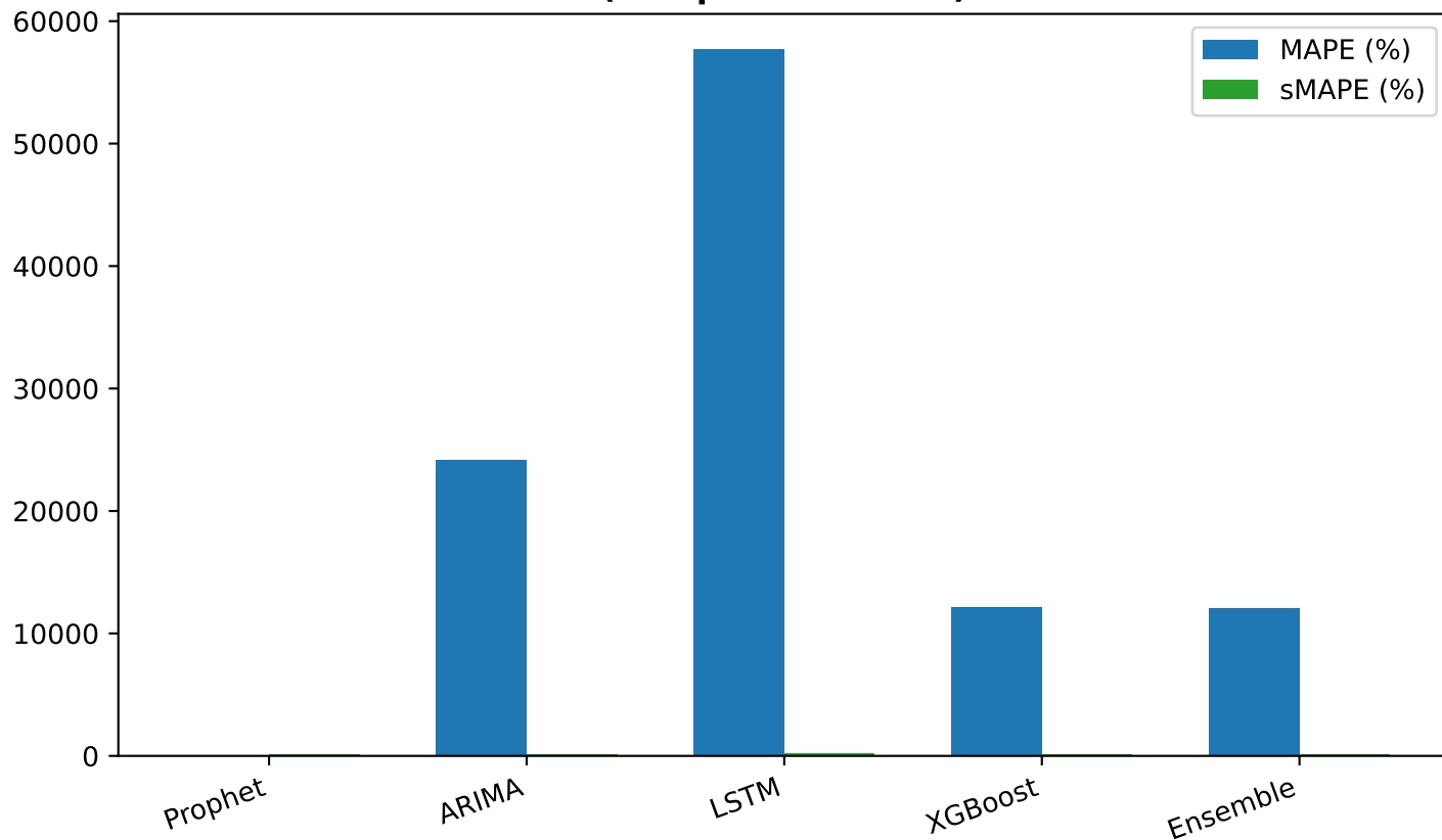
Sai số Tương đối - Mã: 29.L1.3060.FPH3621(D,V) (Vô địch: Ensemble)
