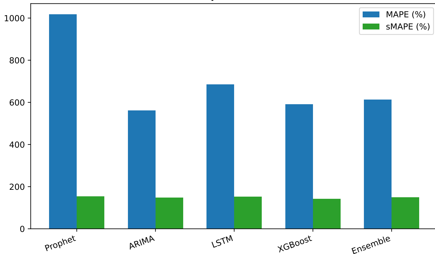
Sai số Tương đối - Mã: 10.L1.8080.589(1-9) (Vô địch: XGBoost)
