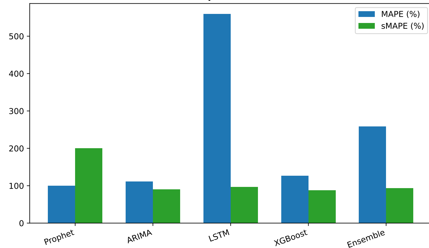
Sai số Tương đối - Mã: 29.L1.3060.FC3619(T) (Vô địch: XGBoost)
