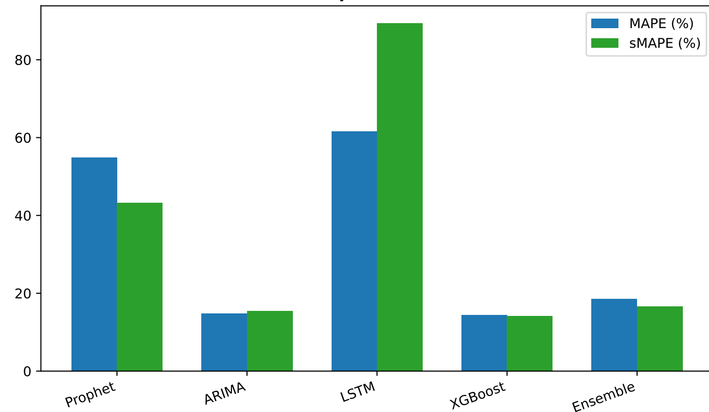
Sai số Tương đối - Mã: 31.L1.LEO-100100-0xx (Vô địch: XGBoost)
