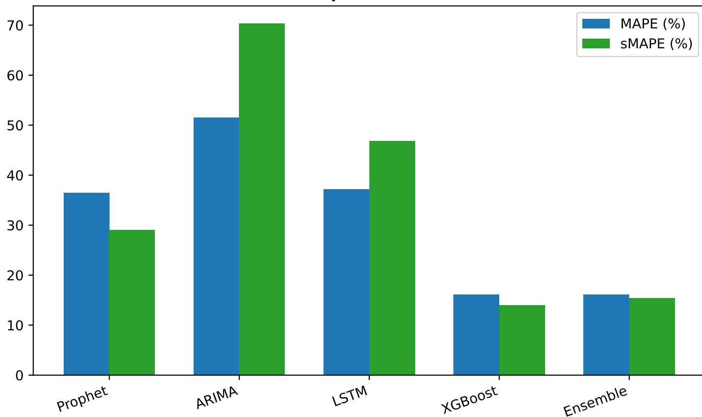
Sai số Tương đối - Mã: 21.C100.DG.(MPECO,MPSET).00 (Vô địch: XGBoost)
