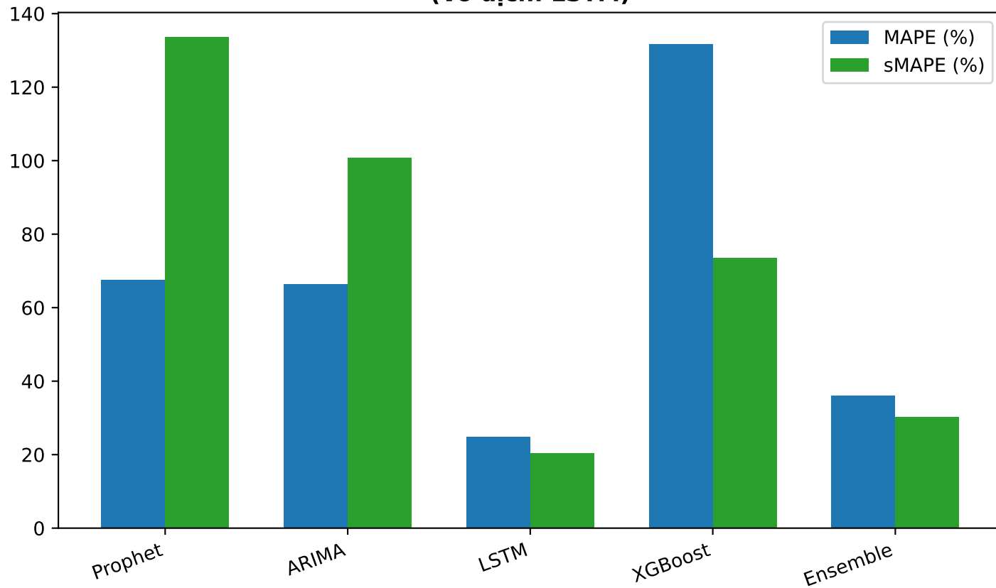
Sai số Tương đối - Mã: 14.L1.3060.US36LB907_ (Vô địch: LSTM)
