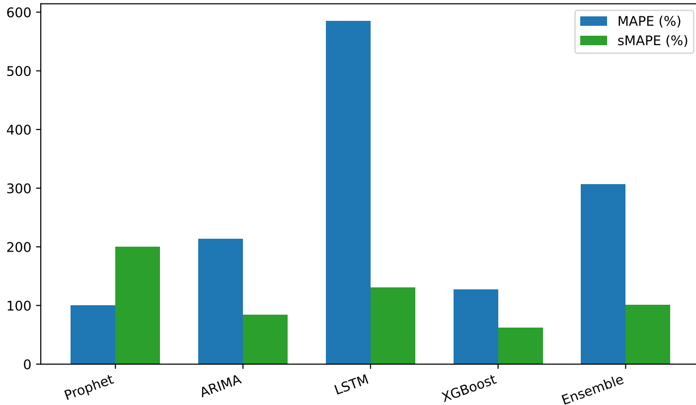
Sai số Tương đối - Mã: 09.L1.6060.CA05GM6601 (Vô địch: XGBoost)
