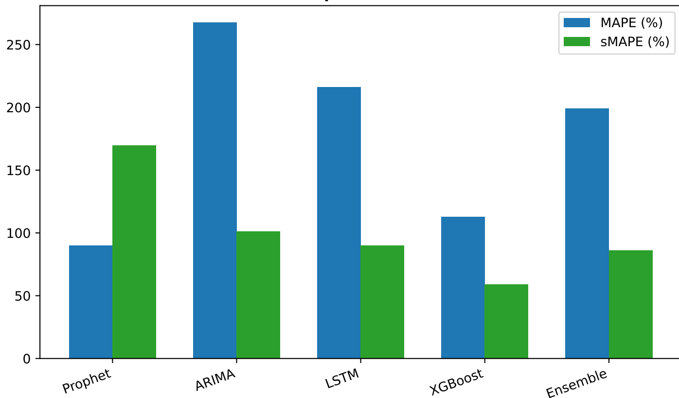
Sai số Tương đối - Mã: 12.L1.2550.250(1-5) (Vô địch: XGBoost)
