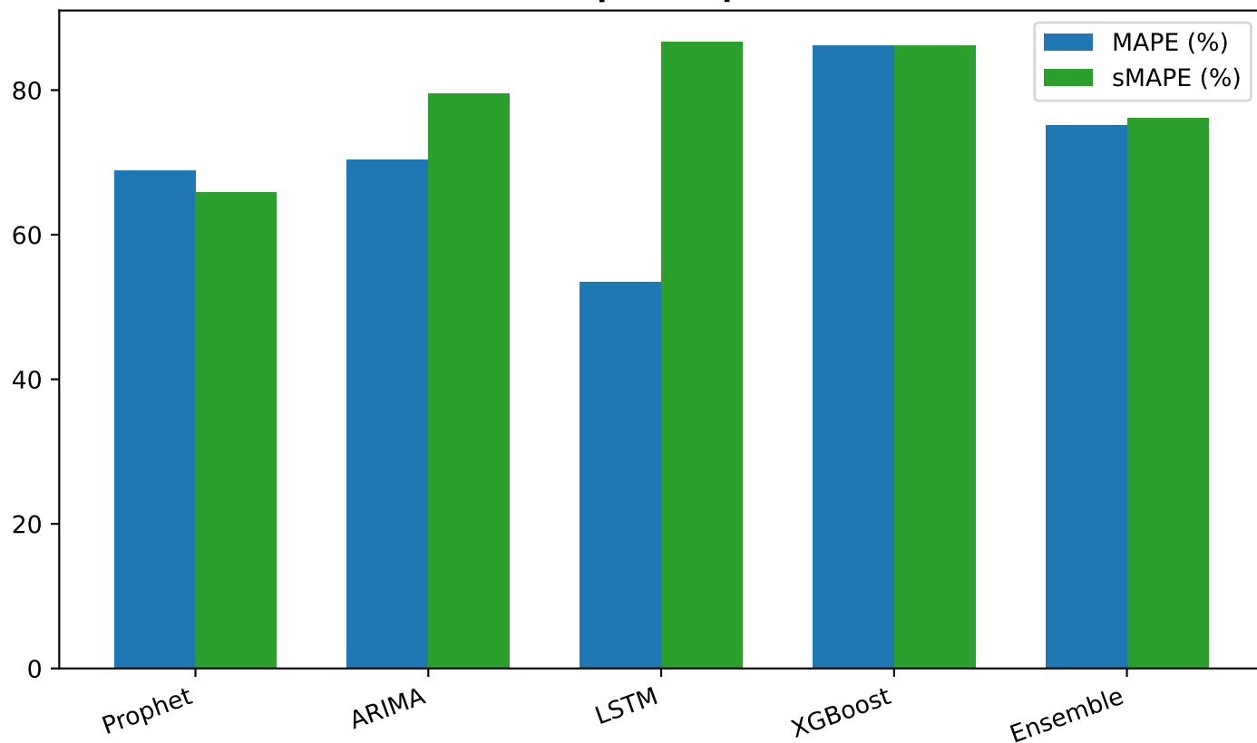
Sai số Tương đối - Mã: 32.L1.ACC-(080160-00x,120120-00x) (Vô địch: Prophet)
