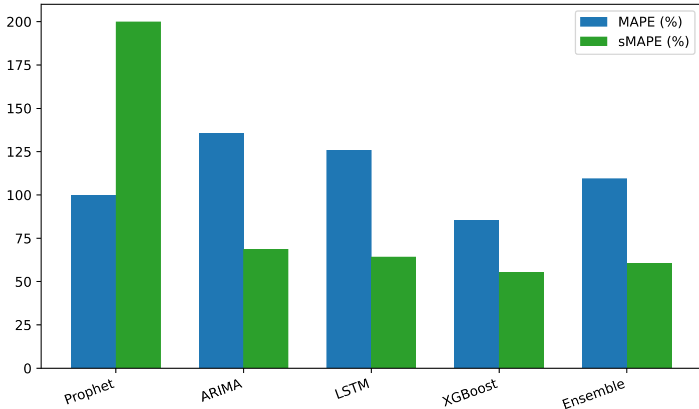
Sai số Tương đối - Mã: 29.L1.3060.FC3623(D,V) (Vô địch: XGBoost)
