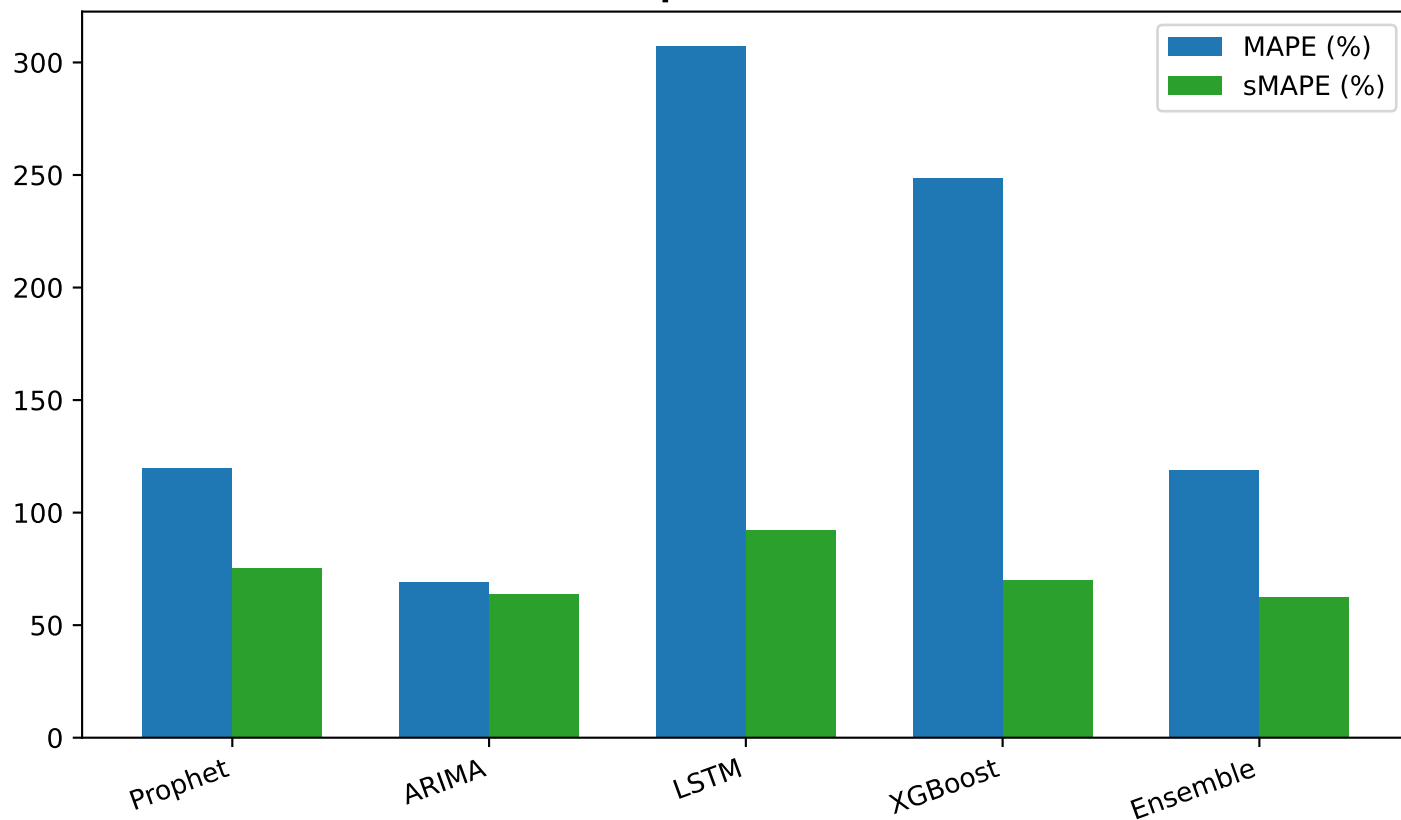
Sai số Tương đối - Mã: 14.L1.3030.334(08,11,18) (Vô địch: Ensemble)
