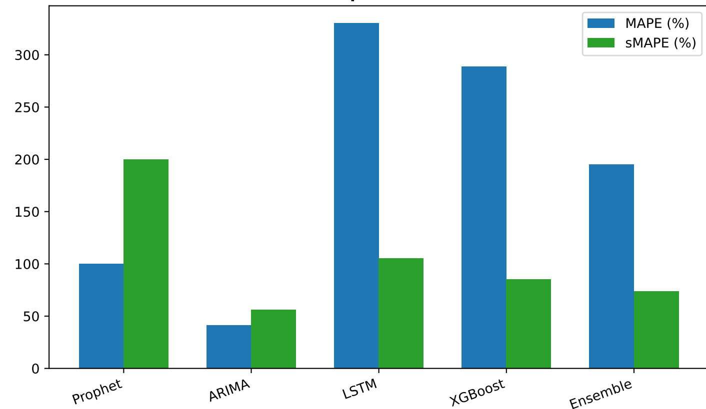
Sai số Tương đối - Mã: 22.CGIW.CR.JOINT.00 (Vô địch: ARIMA)
