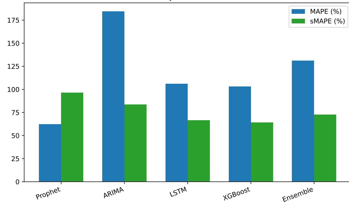
Sai số Tương đối - Mã: 20.L1.6060.86301 (Vô địch: XGBoost)
