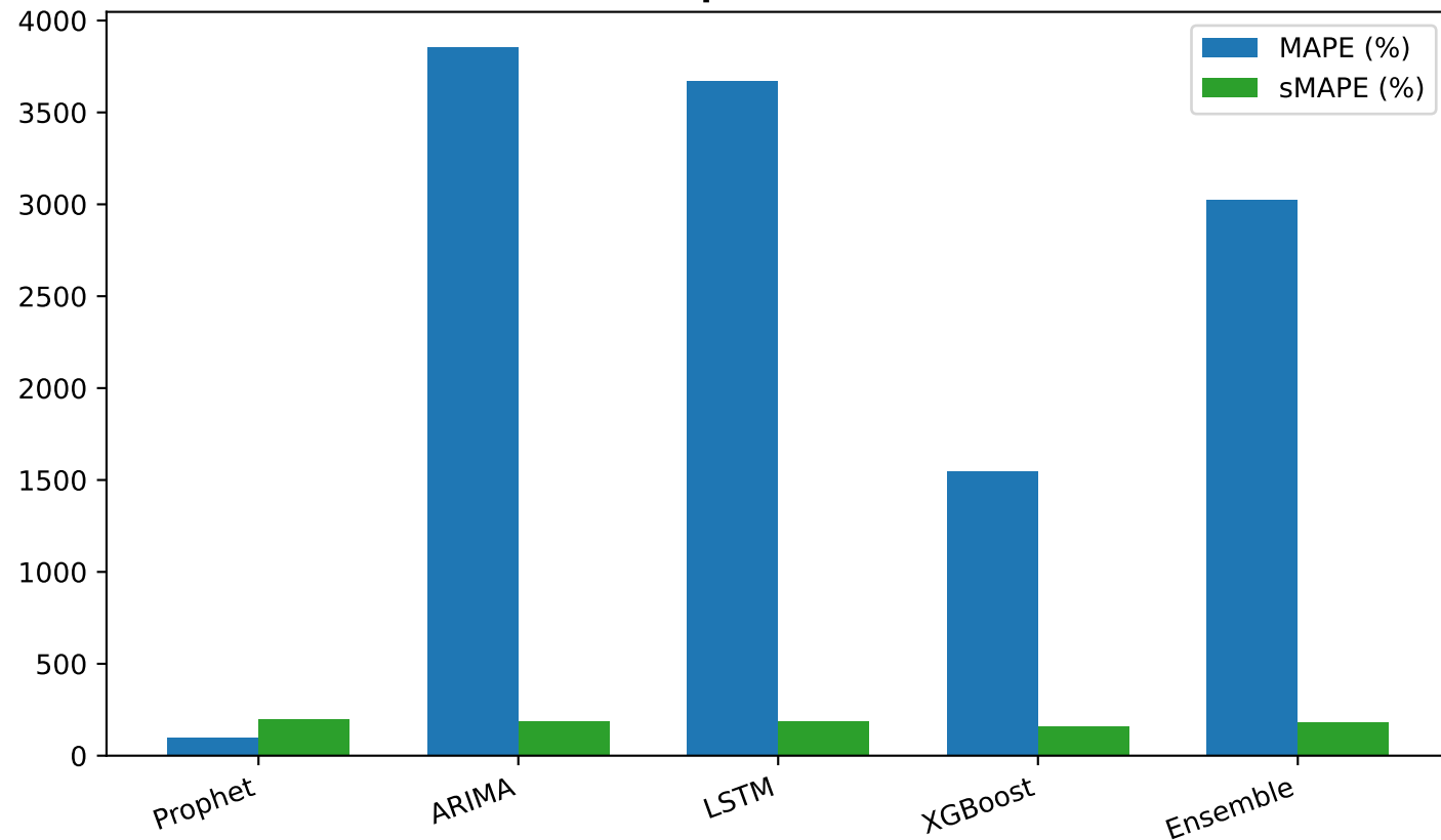
Sai số Tương đối - Mã: 29.L1.3030.F3(05,08,15,17) (Vô địch: XGBoost)
