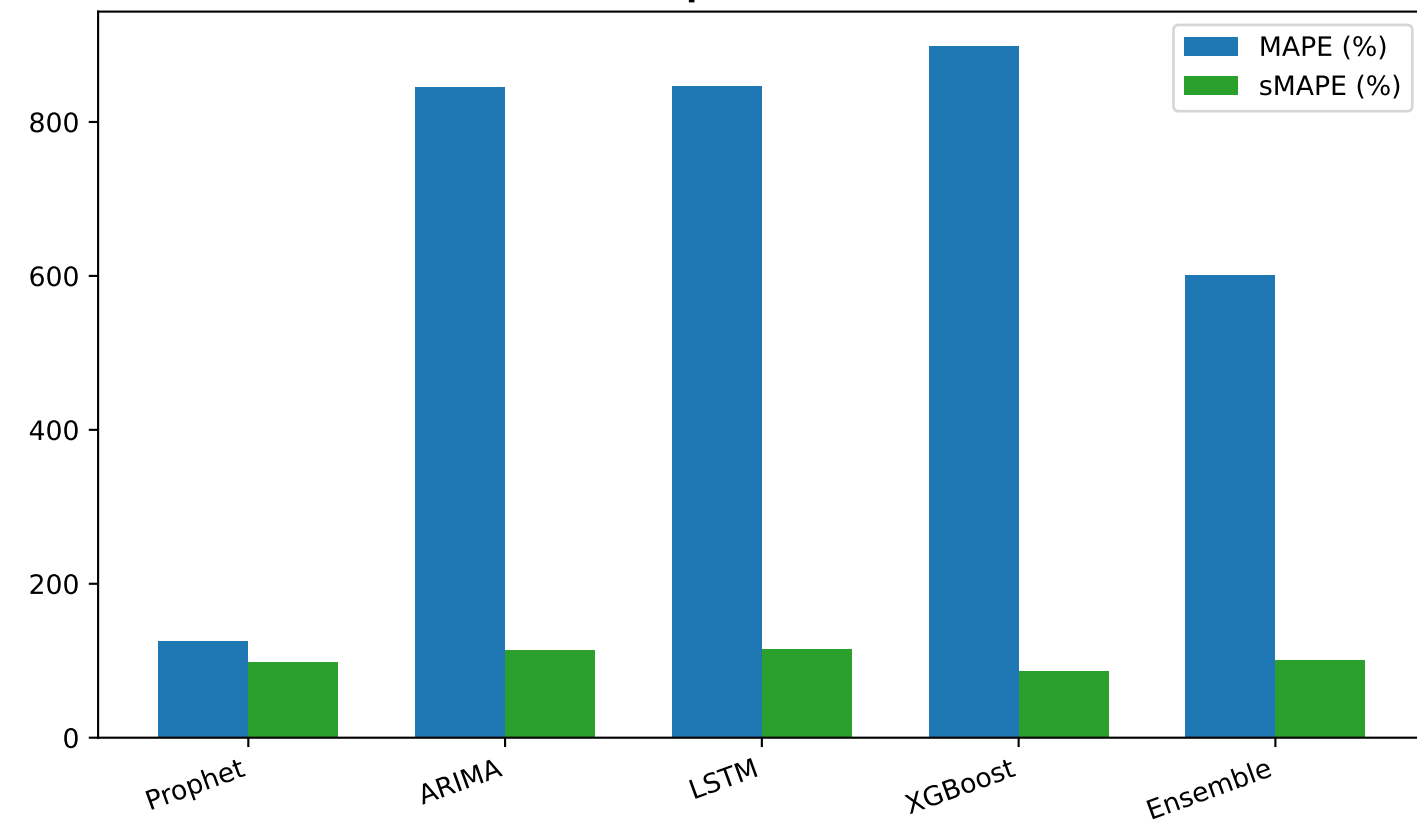
Sai số Tương đối - Mã: 14.L1.3060.US36AG901(D) (Vô địch: XGBoost)
