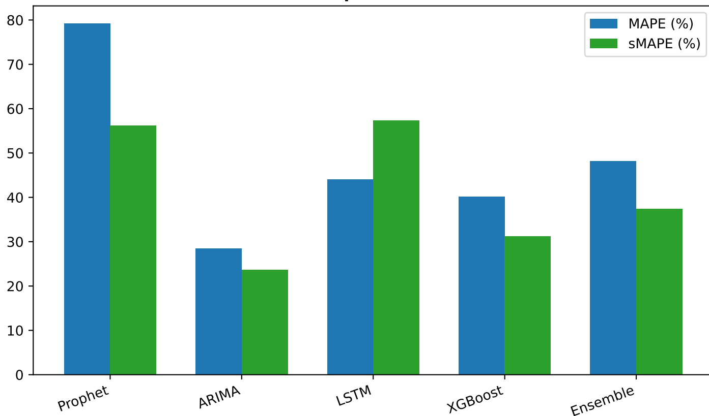
Sai số Tương đối - Mã: 00.KCB.X.NS (Vô địch: ARIMA)
