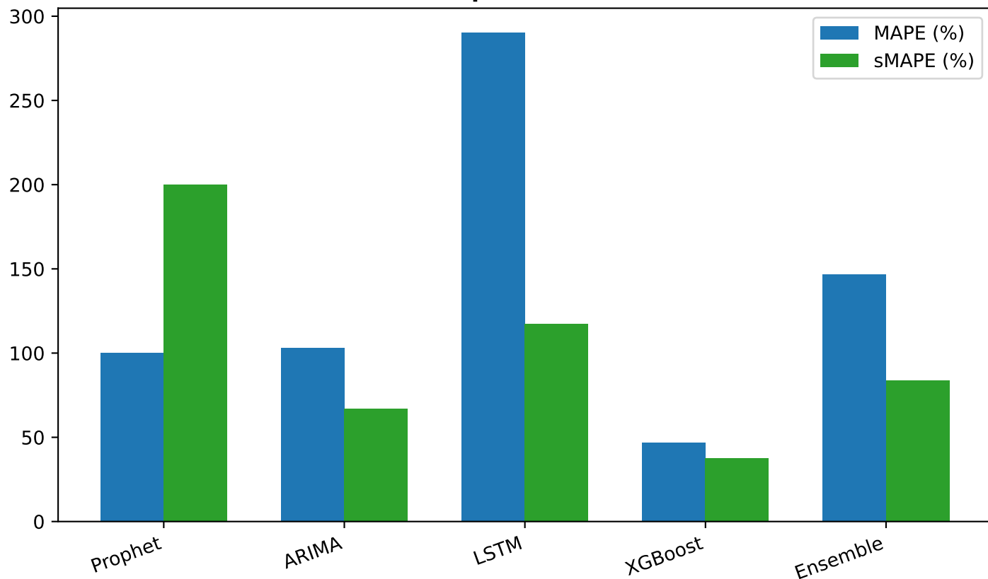
Sai số Tương đối - Mã: 12.L1.2550.U25(18-40) (Vô địch: XGBoost)
