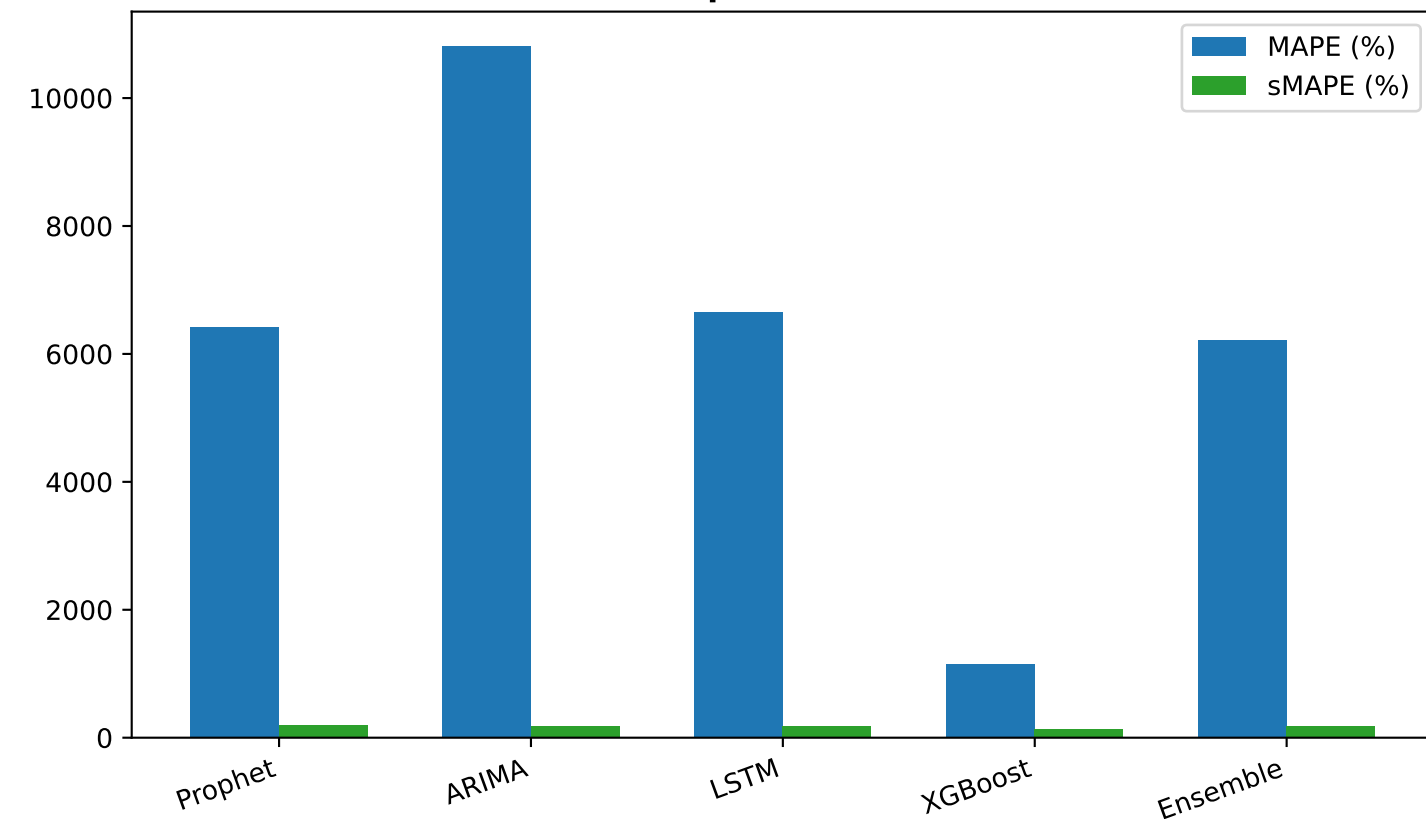
Sai số Tương đối - Mã: 29.L1.6060.FP(6602-6605) (Vô địch: XGBoost)
