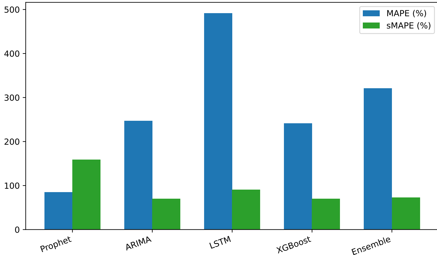
Sai số Tương đối - Mã: 14.L1.3060.A36800(D,V) (Vô địch: XGBoost)
