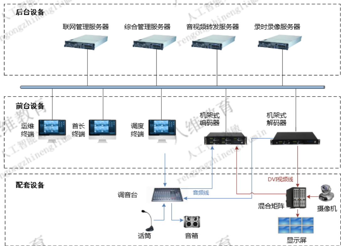
视音频指挥系统构成及工作示意图
