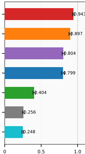
P@10
