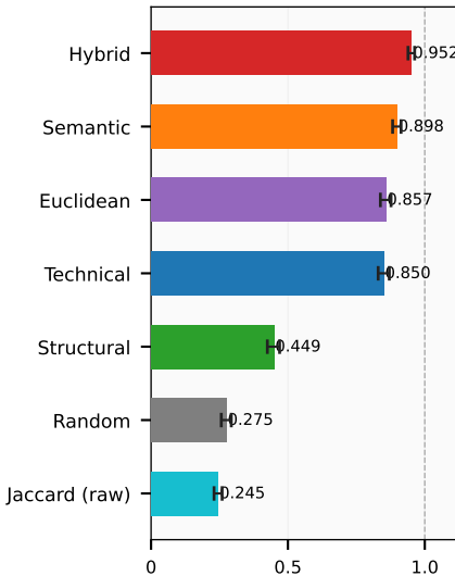
P@3
