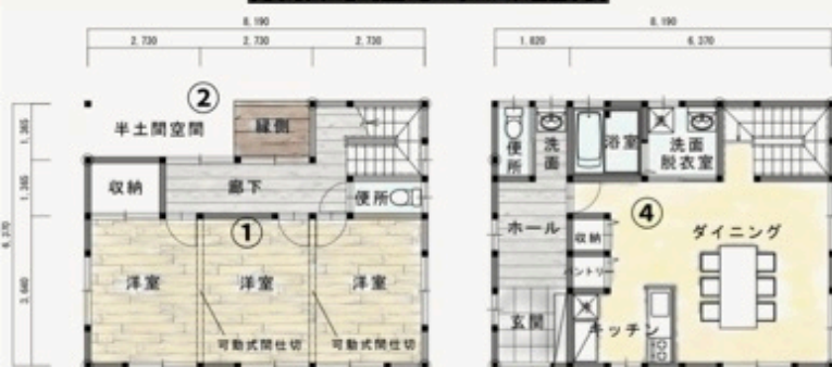
1階平面図 S=1:100
