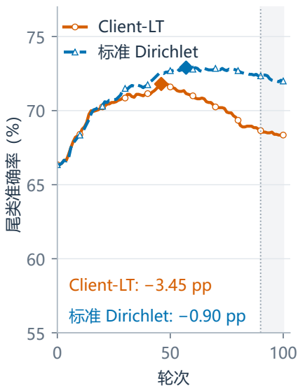
(b) 已有能力 仍会回落
