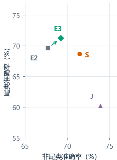
(c) 适当更新 两方面均可改善
