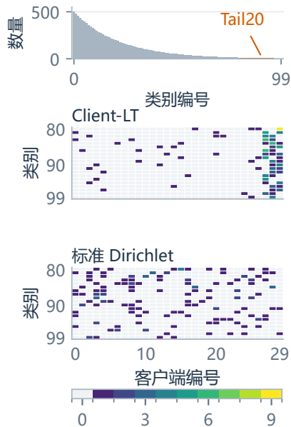
(a) 数量相同 分布不同
